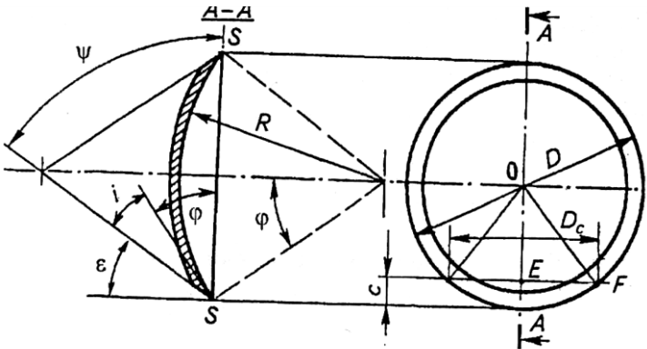
Рисунок 1 – Основные параметры диска
