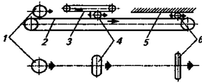
Рис. 16. Схема ленточной прокатывающей машины
