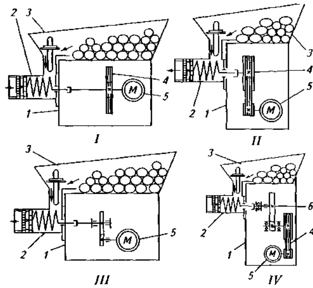
Рис. 6. Кинематические и принципиальные схемы мясорубок
