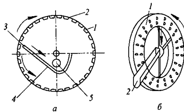
Рис. 12. Схемы цилиндрического и дискового триеров
