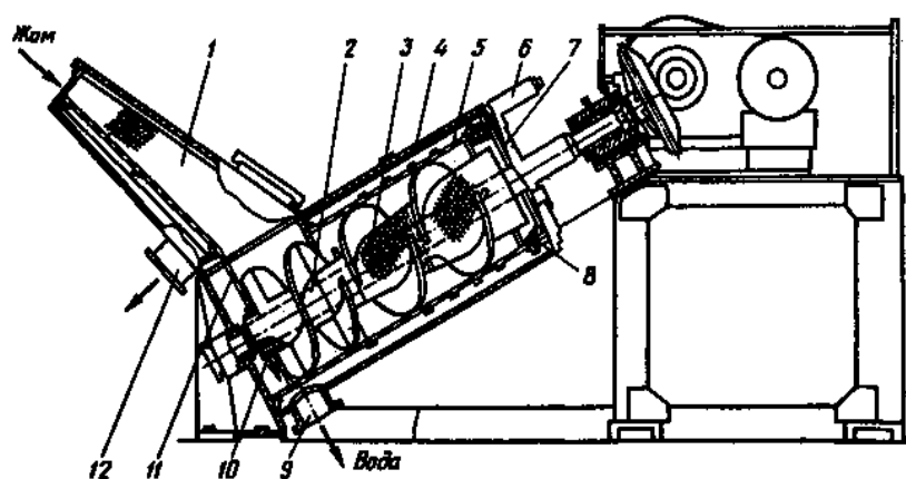
Рис. 14. Схема наклонного отжимного пресса
