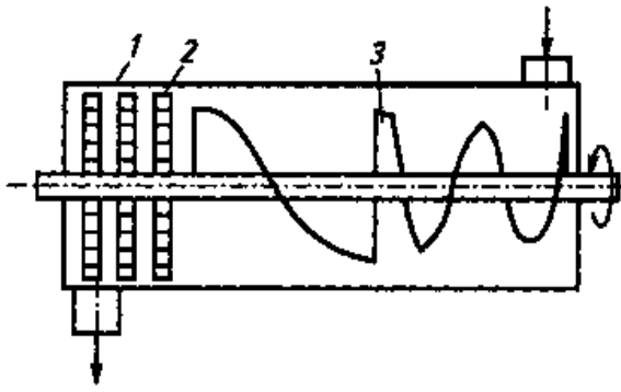
Рис. 5. Схема смесителя непрерывного действия
