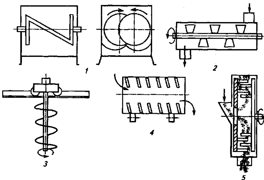
Рис. 19. Схемы смесителей сыпучих продуктов
