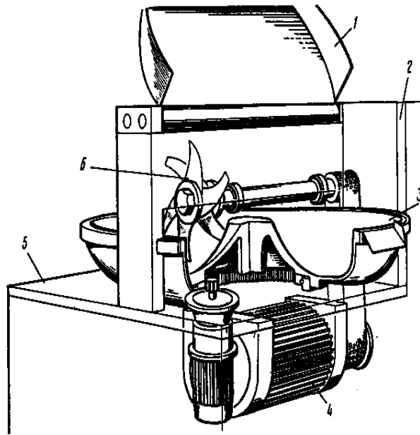
Рис. 5. Куттер
