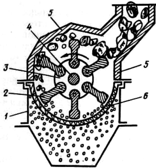
Рис. 3. Схема молотковой дробилки
