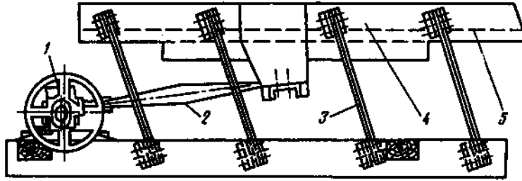
Рис. 10. Качающийся грохот
