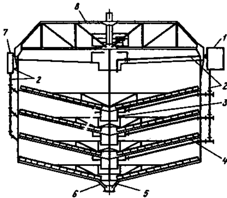
Рис. 10. Многоярусный отстойник
