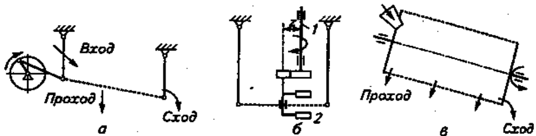
Рис. 9 Схемы рассеивающих машин
