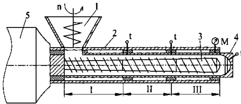
Рис. 17. Схема одношнекового экструдера
