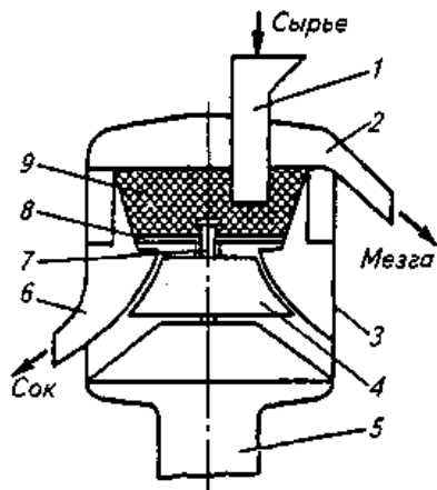
Рис.7. Измельчающая машина для фруктов и ягод
