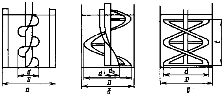
Рис. 3. Схемы мешалок для пластичных масс
