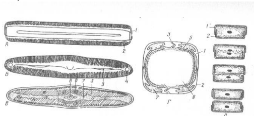
Рис. 8 Диатомовая водоросль пиннулярия ( Pinnularia ): А – вид с пояска; Б – вид со створки; В – продольный разрез, Г – поперечный разрез, Д – вегетативное размножение; 1 – эпитека, 2 – гипотека, 3 – шов, 4 – узелок, 5 – хлоропласт, 6 – пиреноиды, 7 – цитоплазма, 8 – ядро, 9 – вакуоль
