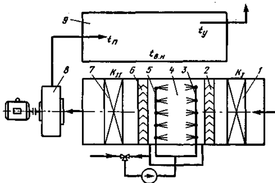
Рис. 18.3 Принципиальная схема прямоточной системы кондиционирования:
