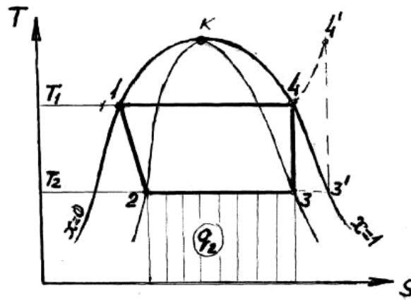
Рис. 8.2. Цикл паровой компрессорной холодильной установки Работа холодильной установки протекает следующим образом.
