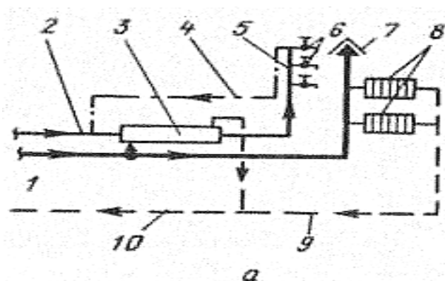
Рис. 17.1. Принципиальная схема параллельного подключения подогревателей к тепловой сети:
