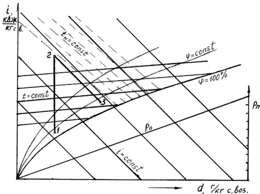
Рис. 6.4. Диаграмма i-d влажного воздуха 1-2 – процесс нагрева; 2-3 – процесс увлажнения
