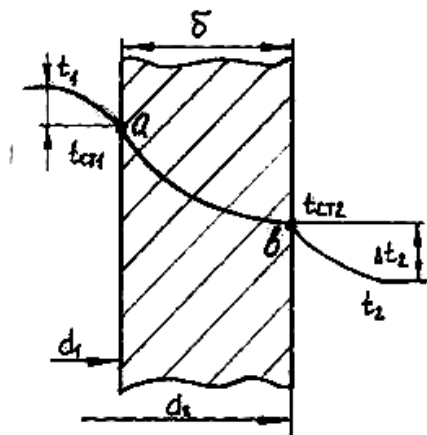
Рис. 13.1. Теплопередача через цилиндрическую стенку
