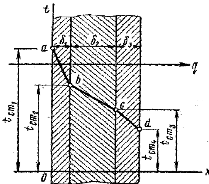
Рис. 10.1. Теплопроводность плоской стенки
