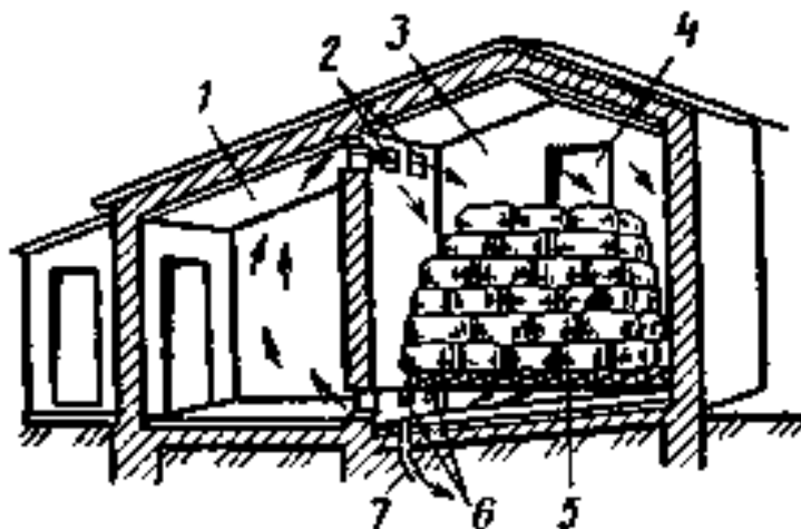
Рис. 21.1. Ледник с боковым расположением льда:
