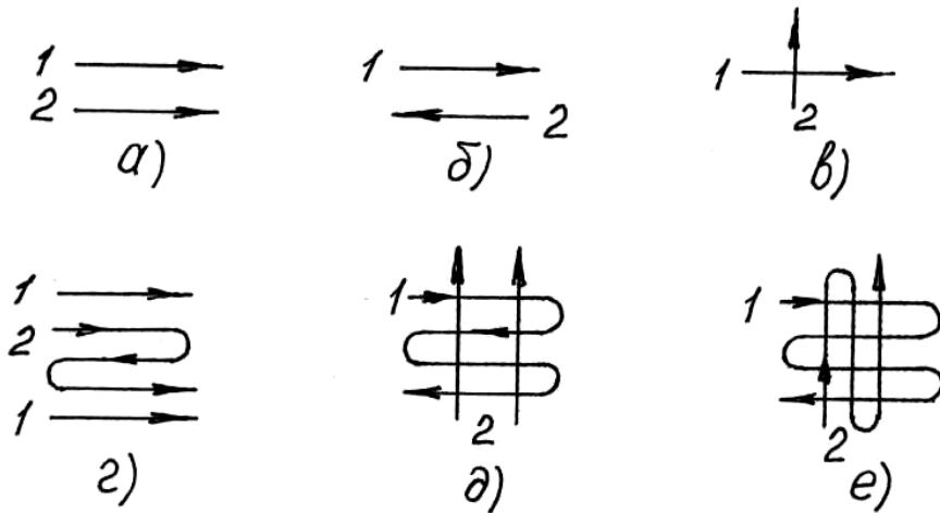
Рис. 13.2. Схемы движения теплоносителей
