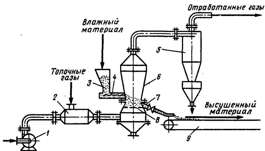
Рис. 20.8. Односекционная сушилка с псевдооживленным слоем:
