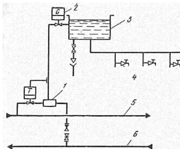
Рис. 17.2. Тупиковая схема системы горячего водоснабжения:
