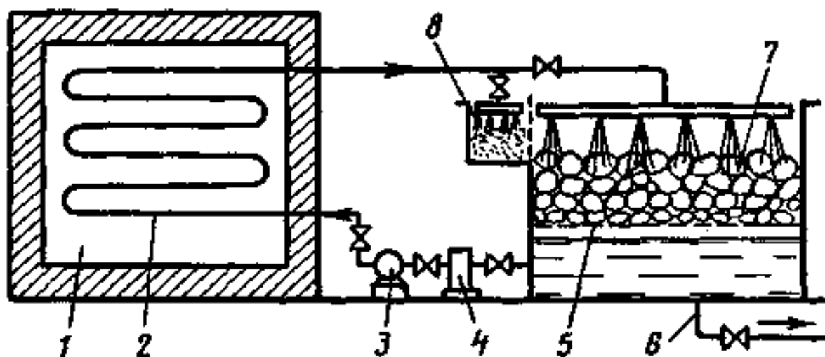
Рис. 21.2. Схема рассольного охлаждения:
