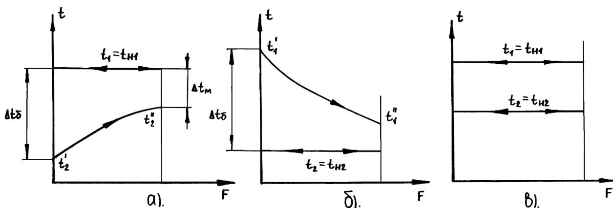
Рис. 13.4. Изменение температуры теплоносителей по поверхности теплообмена при фазовых превращениях теплоносителей:
