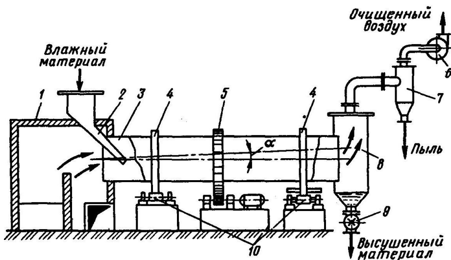
Рис. 20.6. Барабанная сушилка:
