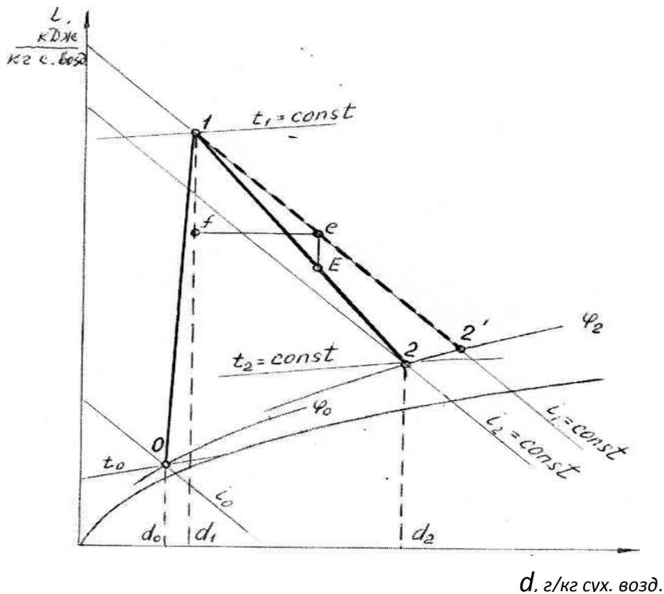
Рис. 20.12. Рабочие процессы в конвективной сушилке на диаграмме i - d воздуха.
