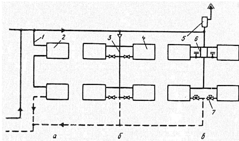
Рис. 16.3. Схема горизонтальной однотрубной системы отопления:
