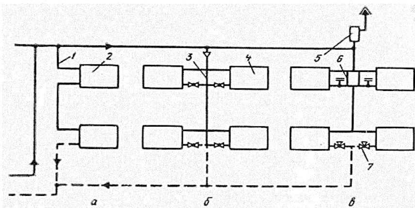
Рис. 16.2. Схема однотрубной системы водяного отопления с верхней разводкой:
