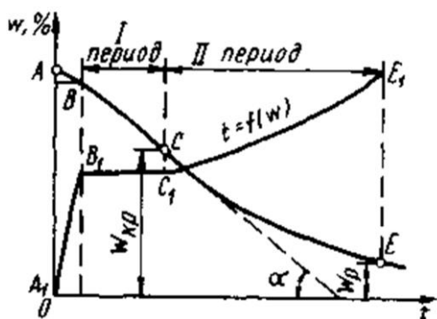
Рис. 20.2. Кривая сушки
