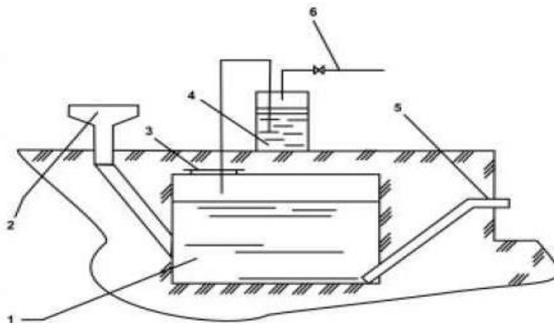
Рис. 20.2. Схема биогазовой установки для фермерского хозяйства;
