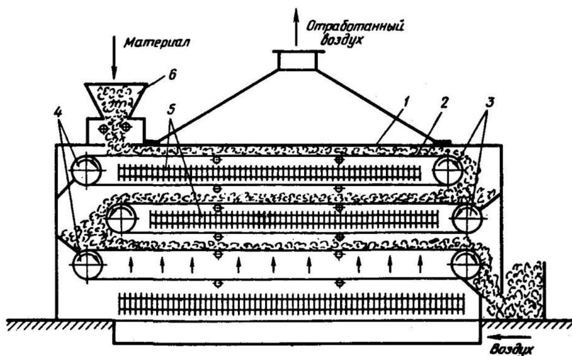
Рис. 20.5. Ленточная сушилка:
