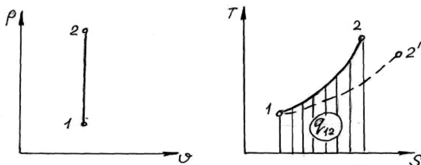
Рис.4.1. Изохорный процесс в координатах p - v и T - s (На рисунке в координатах T - s штриховой линией для сравнения изображен изобарный процесс)
