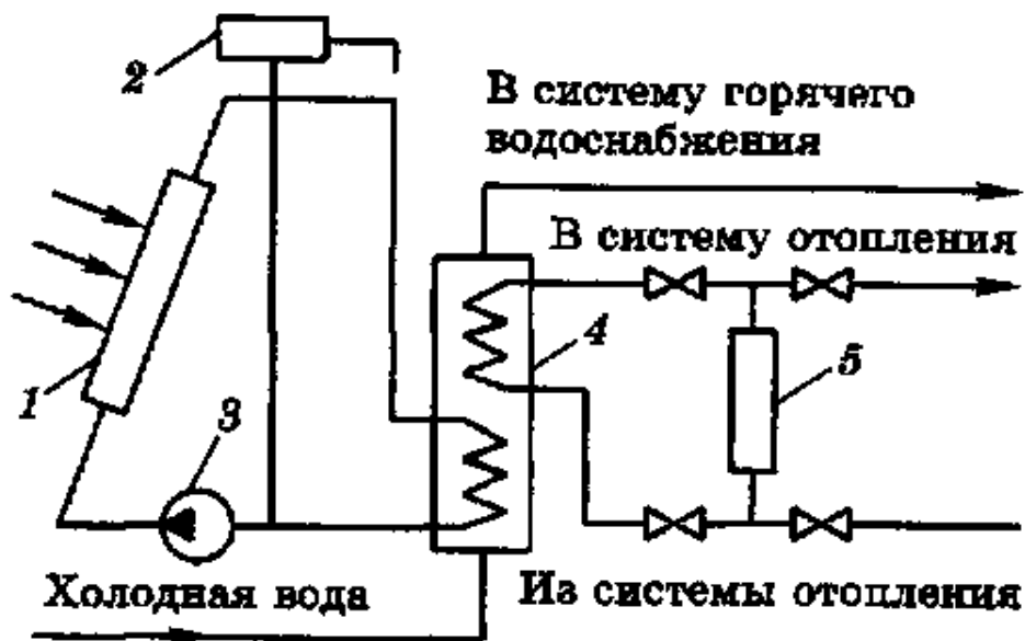
Рис. 20.1. Схема гелиоустановки
