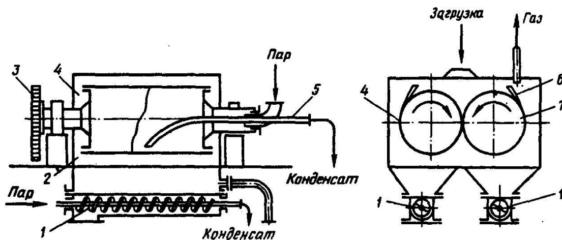
Рис. 20.10. Вальцовая сушилка:
