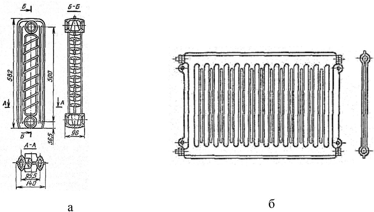
Рис. 16.5. Отопительные радиаторы:
