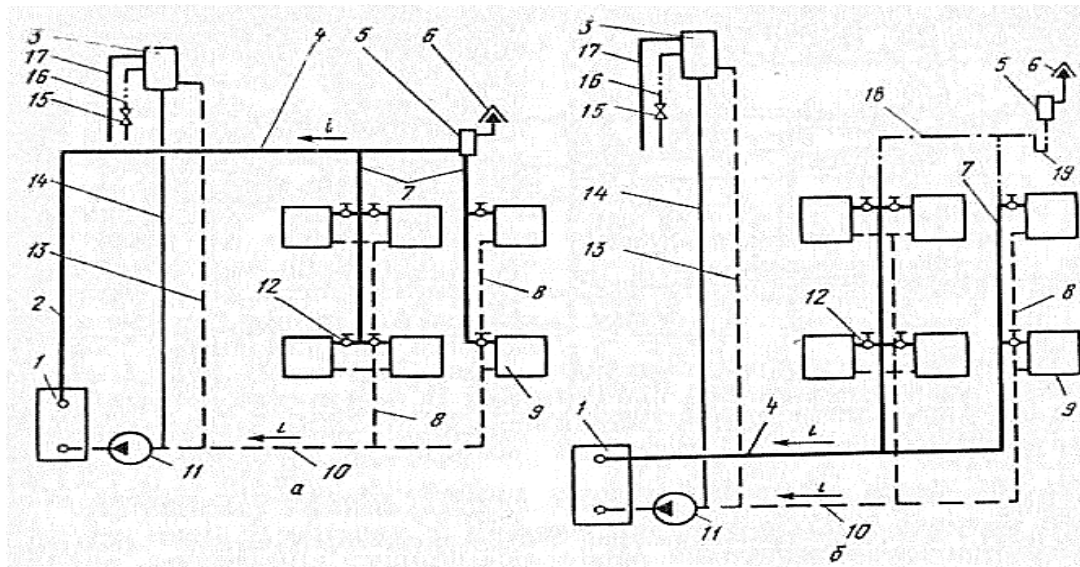
Рис. 16.1. Схемы двухтрубной системы отопления с искусственной циркуляцией:
