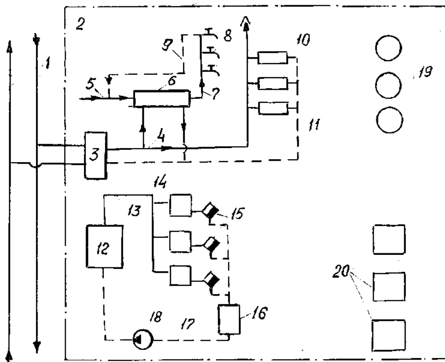
Рис. 1.1. Схема смешанной системы теплоснабжения предприятия:
