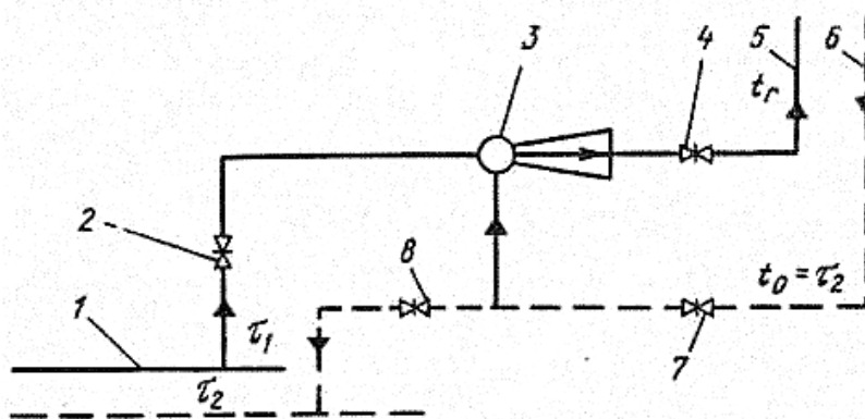
Рис. 16.4. Схема теплового пункта:
