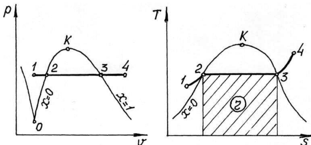
Рис. 6.2. Процесс парообразования в координатах p - v и T - s :
