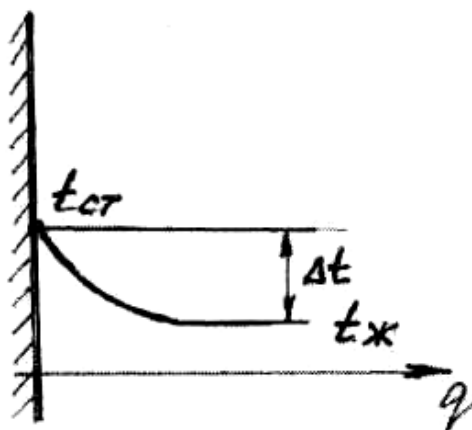
Рис.11.1. Плотность теплового потока при теплоотдаче
