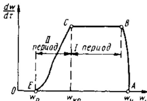
Рис. 20.3. Кривая скорости сушки
