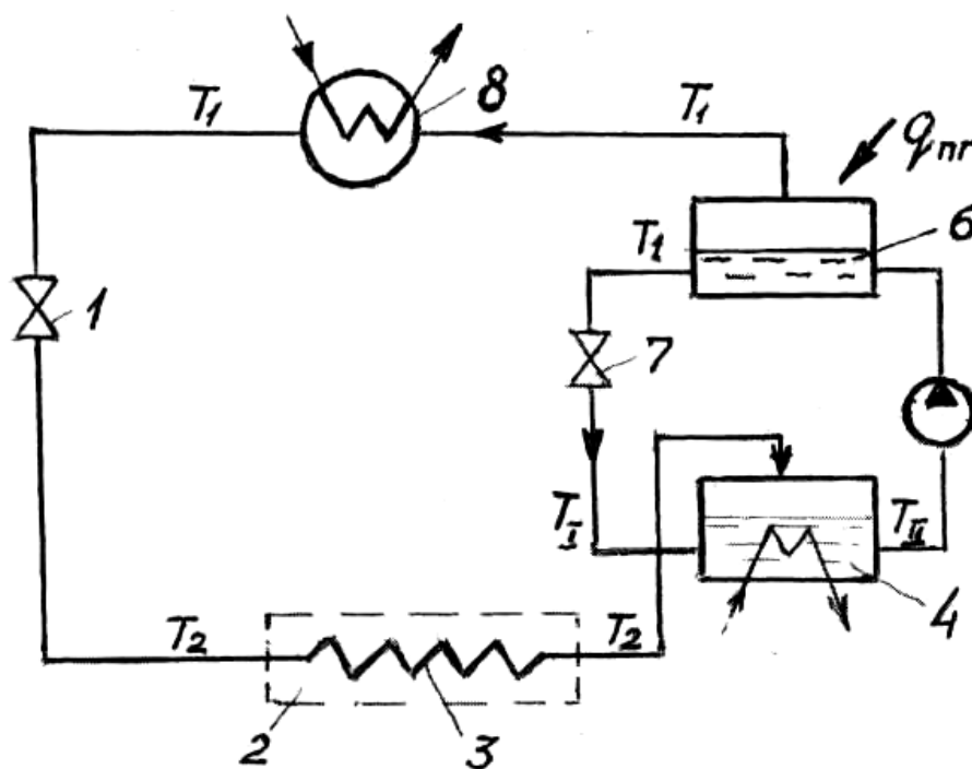
Рис. 8.3. Принципиальная схема абсорбционной холодильной установки
