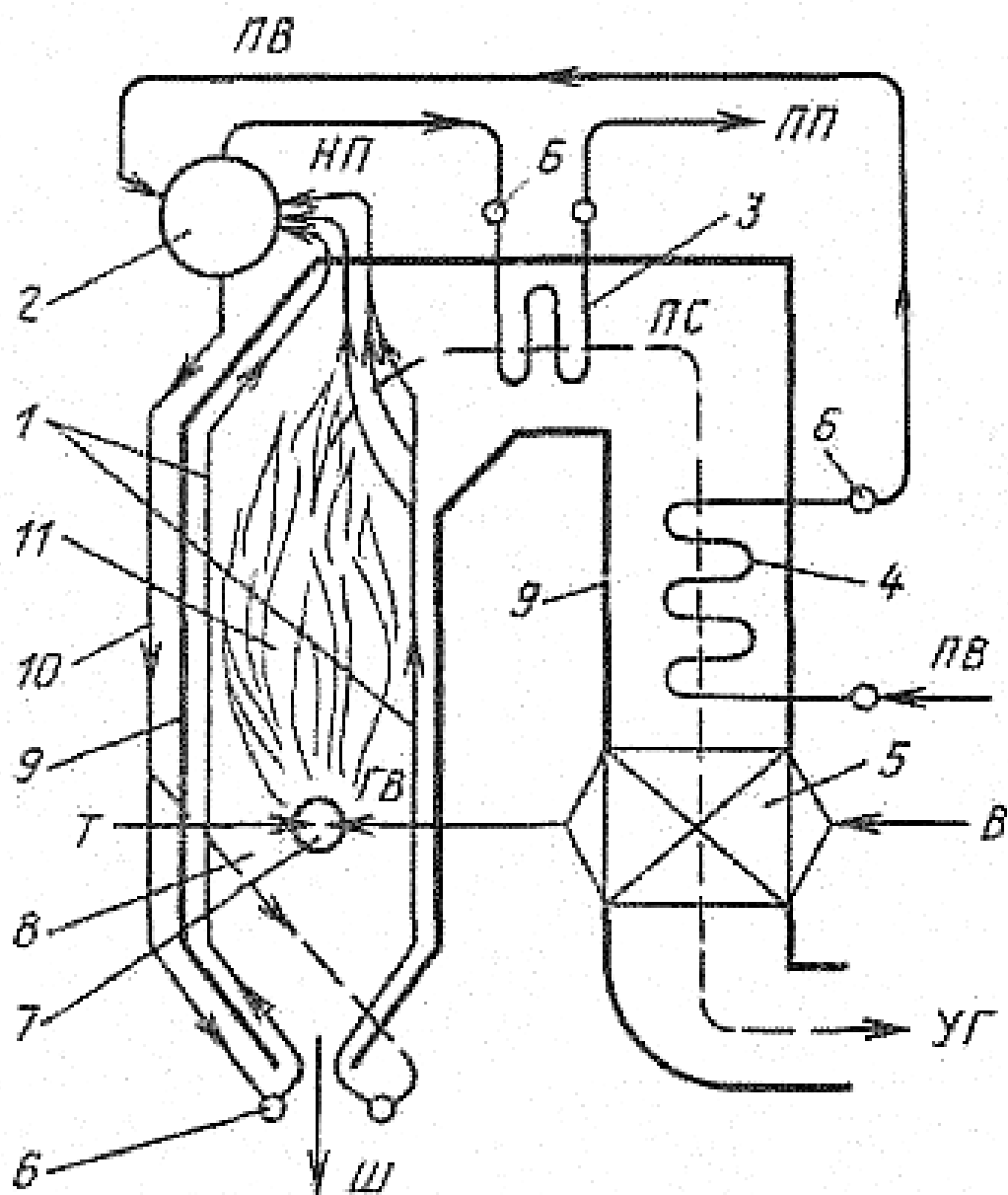
Рис 15.1. Схема вертикально-водотрубного барабанного парового котла с естественной циркуляцией:
