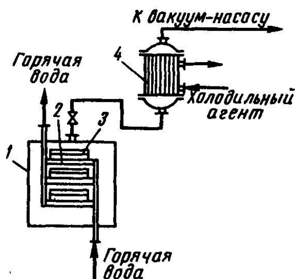
Рис. 20.11. Сублимационная сушилка:
