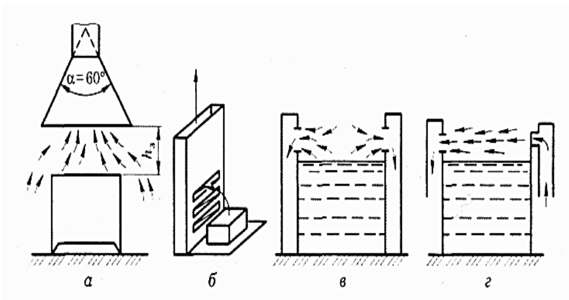
Рис. 18.1. Устройства местной вытяжной вентиляции : а – вытяжной зонт; б – вытяжная панель; в – бортовой отсос, кольцевой; г – бортовой отсос с поддувом.
