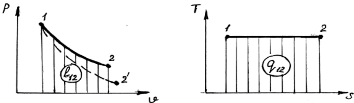
Рис.4.3. Изотермический процесс в координатах p - v и T - s (На рисунке в координатах p - v штриховой линией для сравнения изображен адиабатный процесс)
