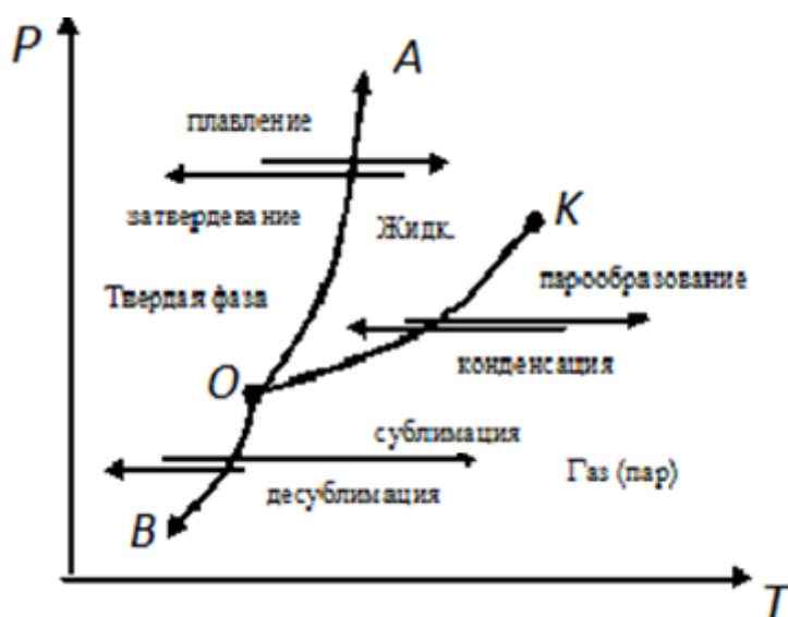
Рис. 6.1. Диаграмма фазовых переходов
