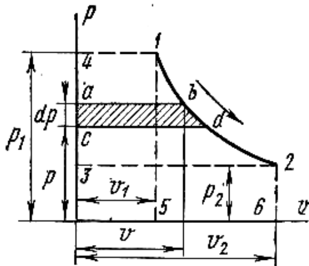
Рис. 7.1. К определению располагаемой работы
