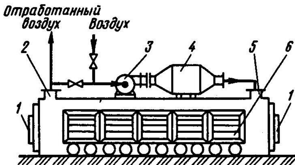
Рис. 20.4. Туннельная сушилка:
