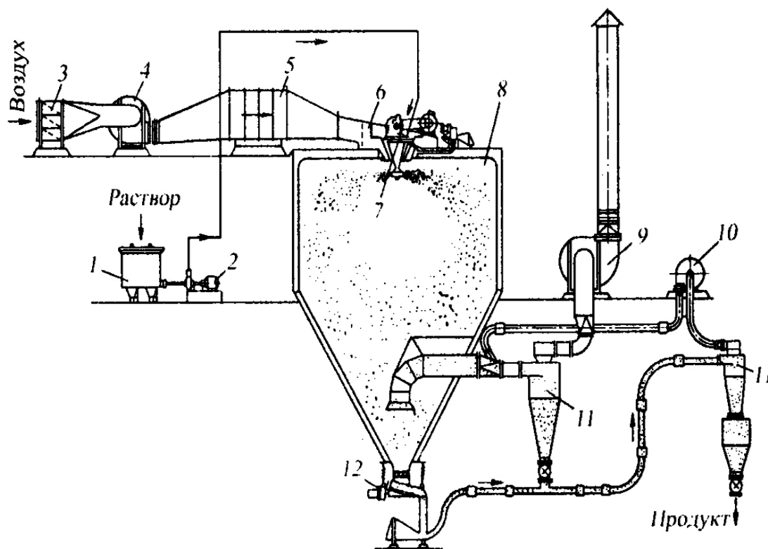
Рис. 20.9. Схема распылительной дисковой сушилки:
