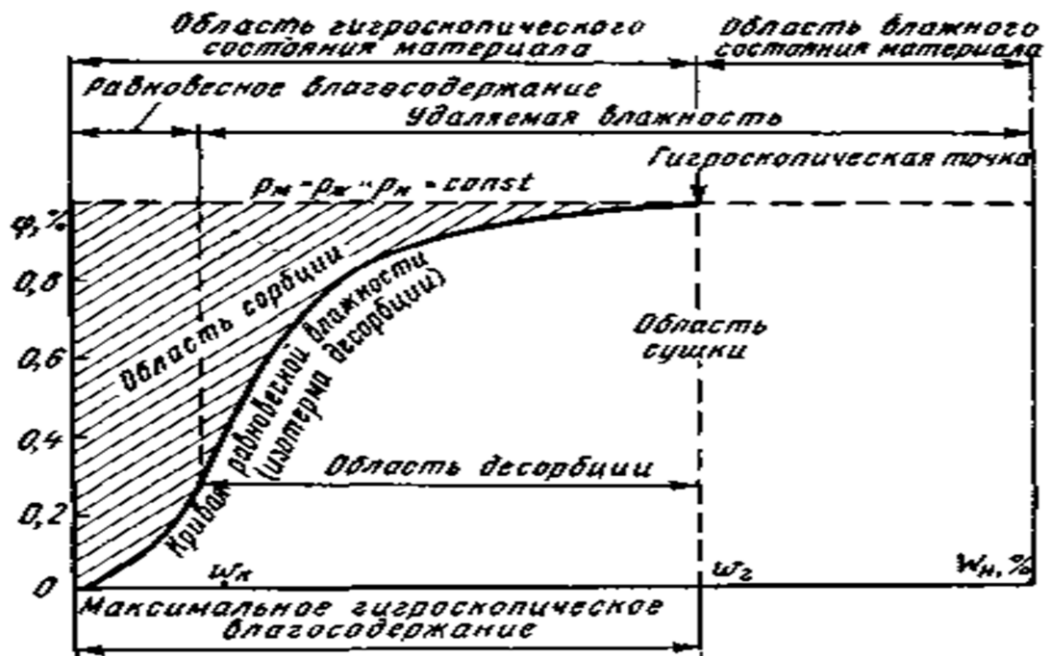
Рис. 20.1. Изотерма сорбции-десорбции капиллярно-пористых тел
