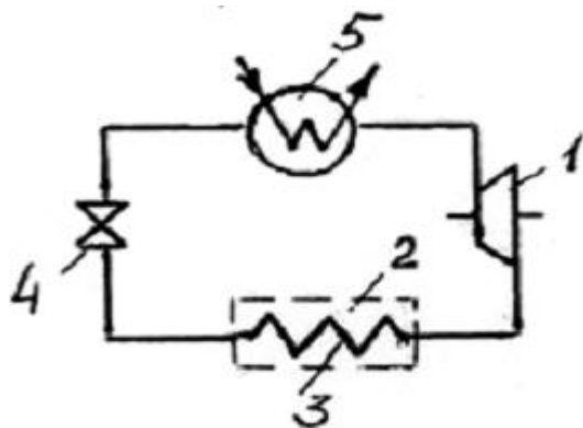
Рис. 8.1. Принципиальная схема паровой компрессорной холодильной установки
