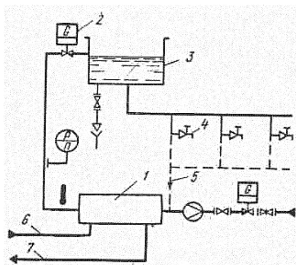
Рис. 17.3. Схема системы горячего водоснабжения с естественной циркуляцией:
