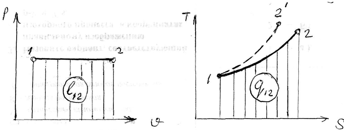
Рис.4.2. Изобарный процесс в координатах p - v и T - s (На рисунке в координатах T - s штриховой линией для сравнения изображен изохорный процесс)
