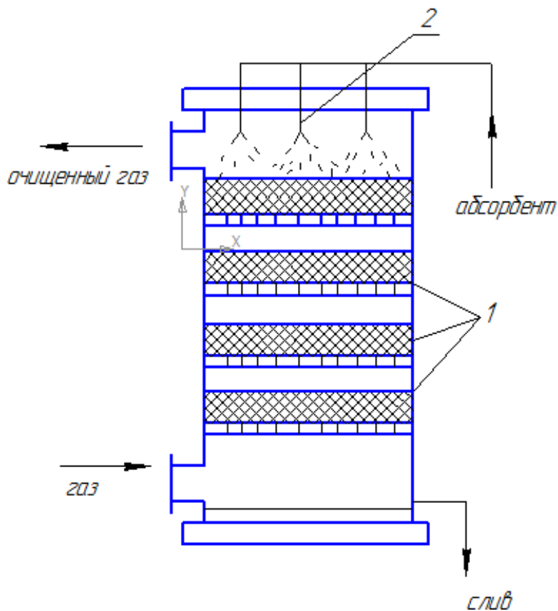
1 – насадки; 2 – разбрызгиватели
