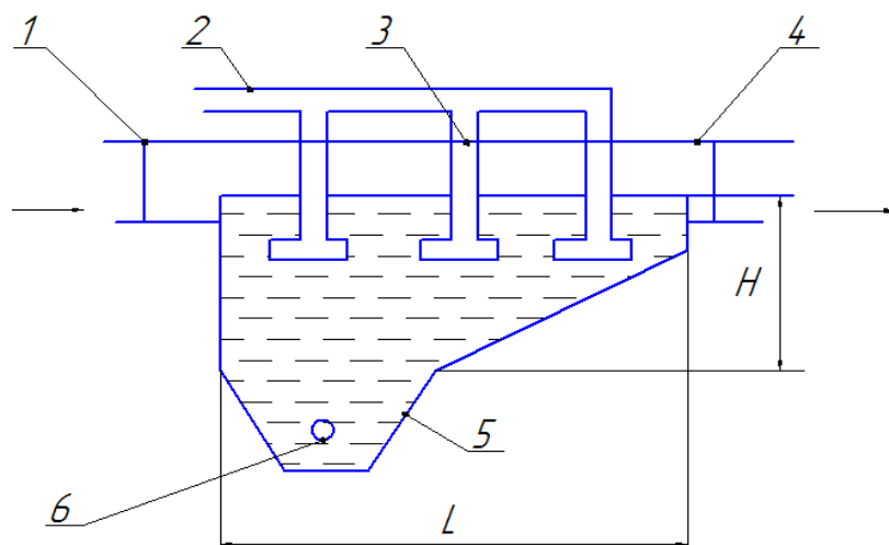
Рисунок 2 – Схема аэрируемой песколовки: 1 – входная труба; 2 – воздуховод; 3 – воздухораспределители; 4 – выходная труба; 5 – шламоборник; 6 – отверстие
