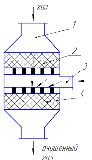
Рисунок 3 – Двухступенчатый каталитический нейтрализатор
