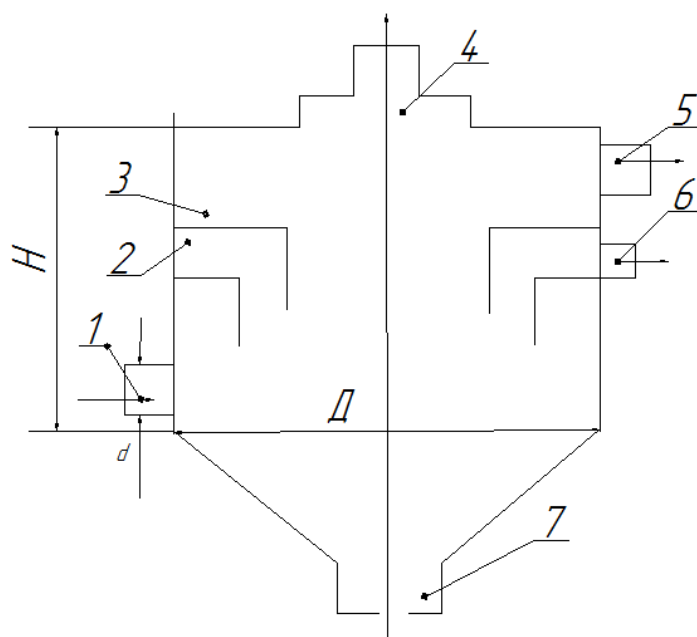
Рисунок 6 – Схема комбинированного гидроциклона: 1 – входной трубопровод; 2 – камера; 3 – приемная камера; 4,5,6 – трубопроводы; 7 – шламособорник.
