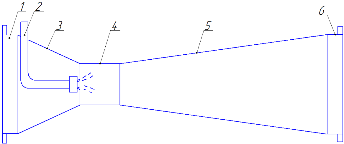
Рисунок 4. – Схема трубы Вентури: 1.6 – входной и выходной патрубки; 2 – форсунка; 3 – конфузур; 4 – горловина; 5 – фиффузор.
