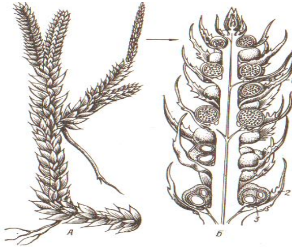
Рис. 13 Селагинелла селоговидная а -общий вид; б - спороносный колосок: 1- микроспорофилл с микроспорангием, 2- мегаспорофилл с мегаспорангием, 3- язычок
