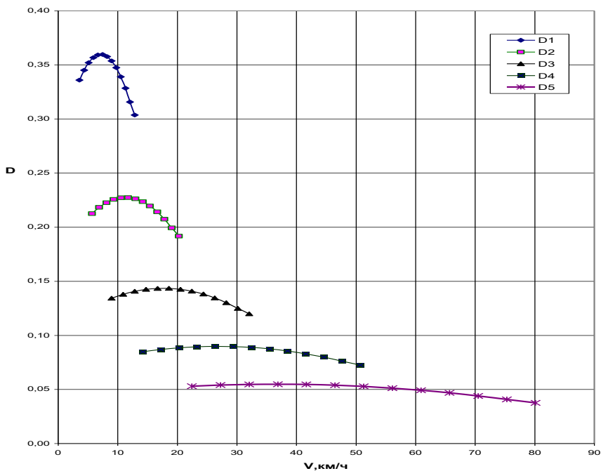
Диаграмма 4 - Динамическая характеристика автомобиля
