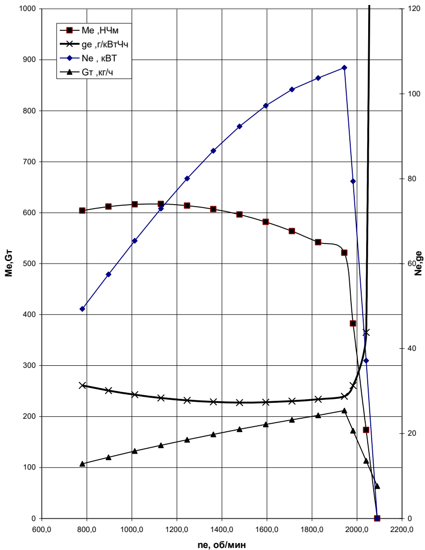
Диаграмма 1 - Регуляторная характеристика дизеля, как функция частоты вращения
