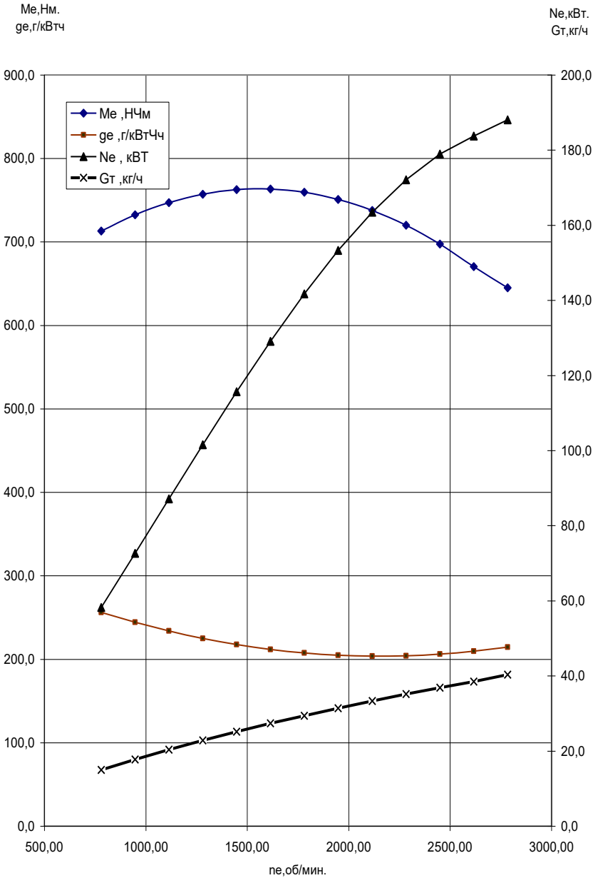
Диаграмма 3 - Скоростная характеристика автомобильного двигателя
