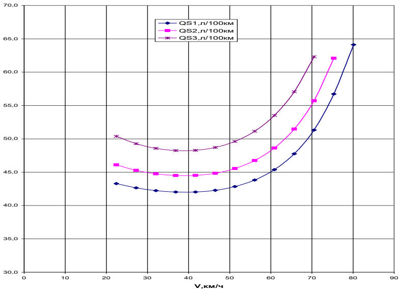
Диаграмма 5 - Экономическая характеристика автомобиля
