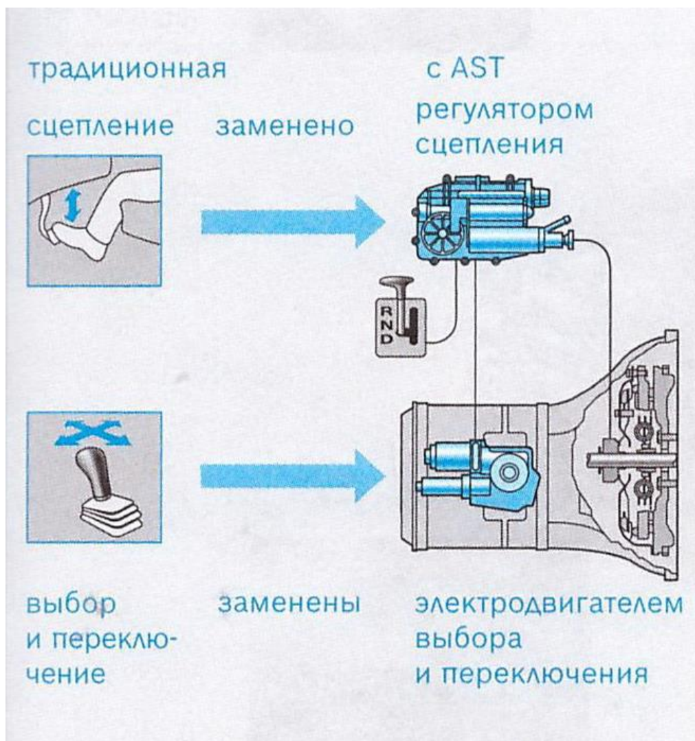
Рисунок 3 – Схема трансформации включения сцепления в РКПП
