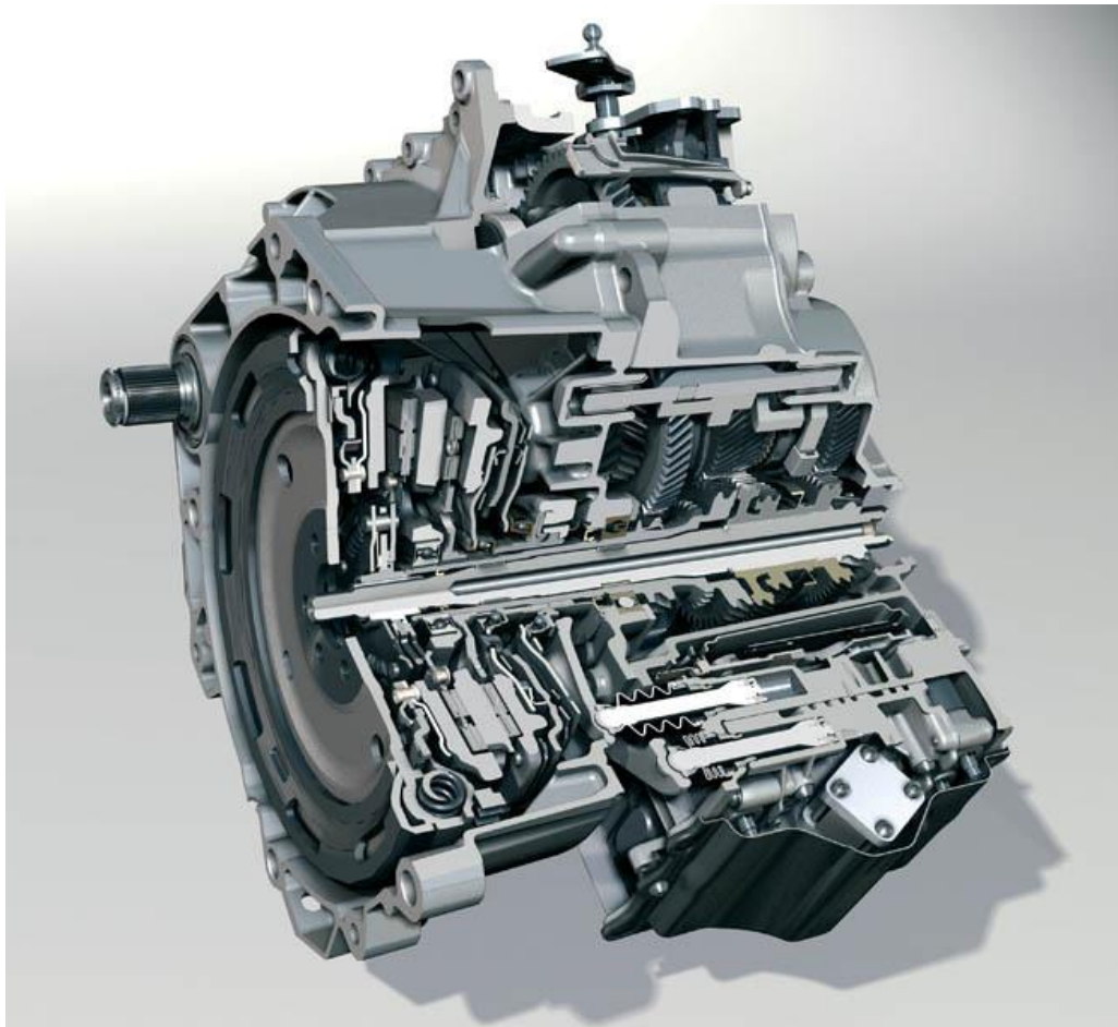
Рисунок 9 – Коробка DSG от Фольксваген
