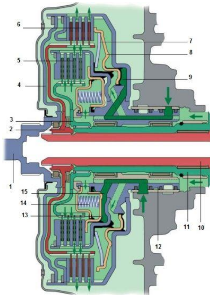
Рисунок 13 – Муфта сцепления мокрого типа:
