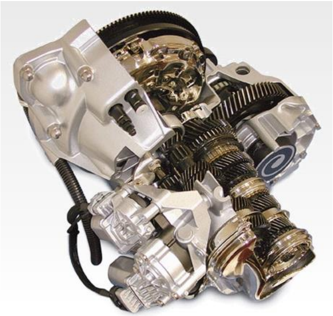
Рисунок 1 - РКПП
