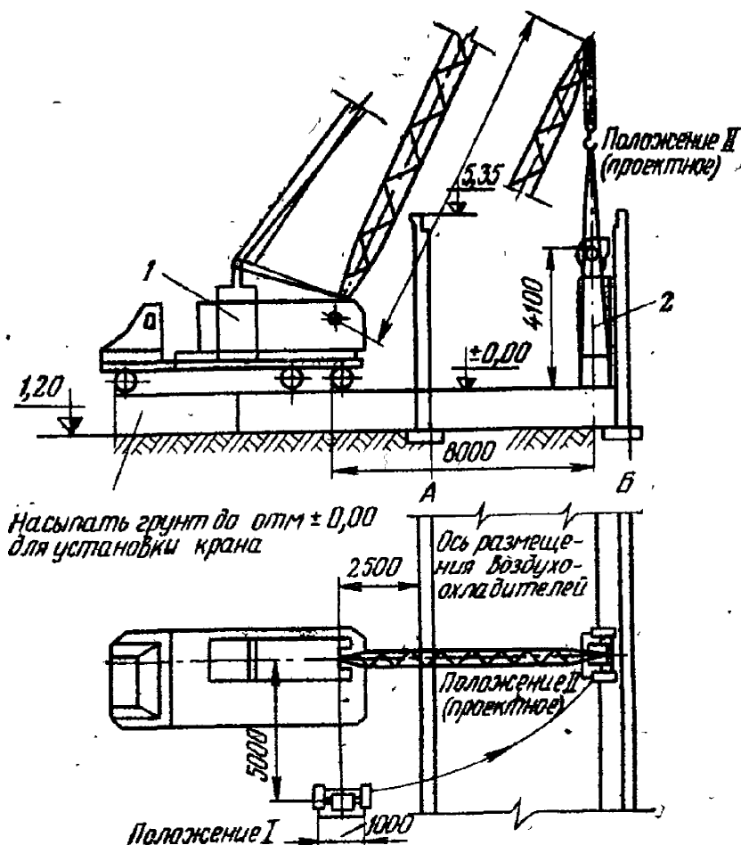
Рис. 5.5. Схема монтажа напольных воздухоохлаждателей поточно-совмещенным способом:
