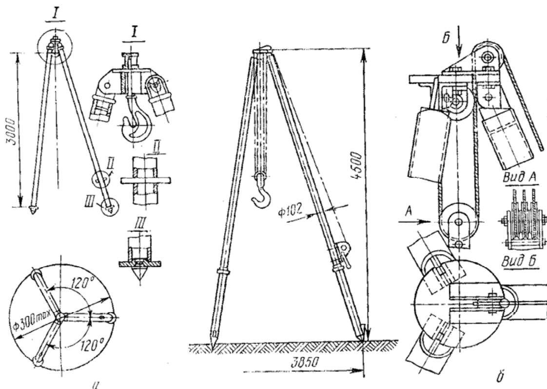
Рис. 1.5. Схема тренога: а - легкий; б - тяжелый
