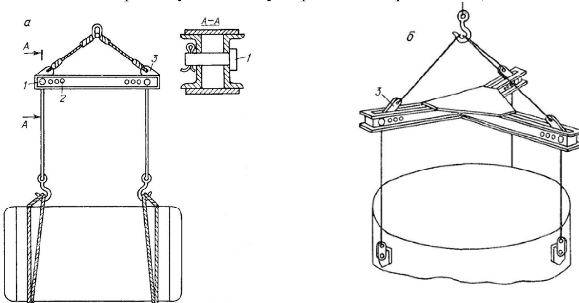
Рис. 1.13. Траверы.
