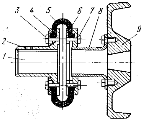
Рис. 4.1. Эластичная муфта: 1 — вал электродвигателя; 2 — полумуфта; 3, 7 — болты; 4 — нажимной диск; 5 — упругий элемент; 6 — диск-проставка; 8 — проставка; 9 — маховик компрессора
