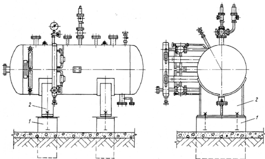
Рис. 6.1. Размещение на фундаменте линейного ресивера: 1 - бетонный фундамент; 2 - металлическая опорная стойка.
