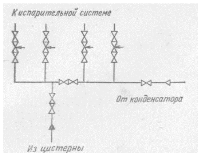
Рис. 9.2. Схема подсоединения аммиачной цистерны при отсутствии центральной регулирующей станции
