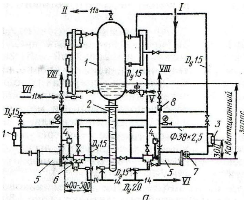
Рис. 8.6. Схема расположения датчиков ПРУ-5:
