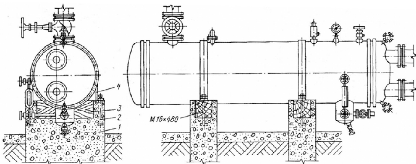
Рис. 5.1. Размещение на фундаменте кожухотрубного конденсатора:
