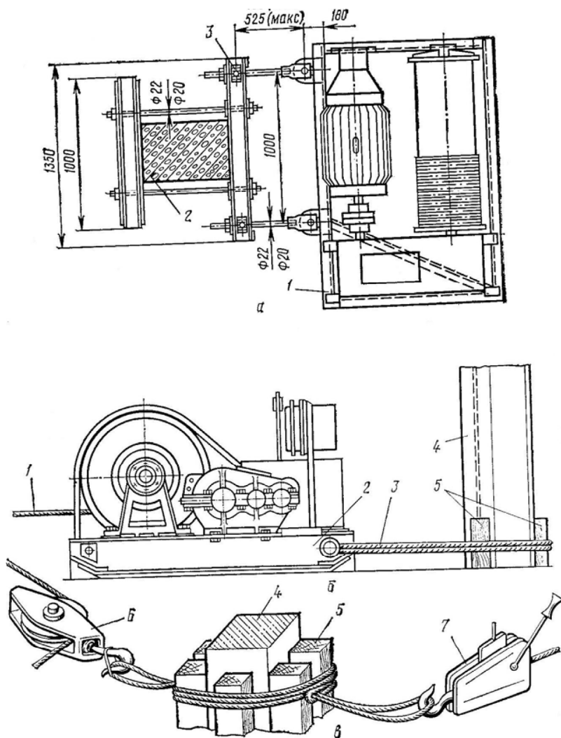
Рис. 1.19. Схемы крепления лебедок к колоннам здания: а - электрической с помощью инвентарного приспособления (1 - рама лебедки; 2 - колонна; 3 - инвентарное приспособление); б - то же, с помощью стального каната; в - ручной рычажной и отводного блока (1 - сбегаящая нитка полиспаста; 2 - рама лебедки; 3 - стальной канат; 4 - колонна; 5 - подкладки; 6 - отводной блок; 7 - рычажная лебедка)
