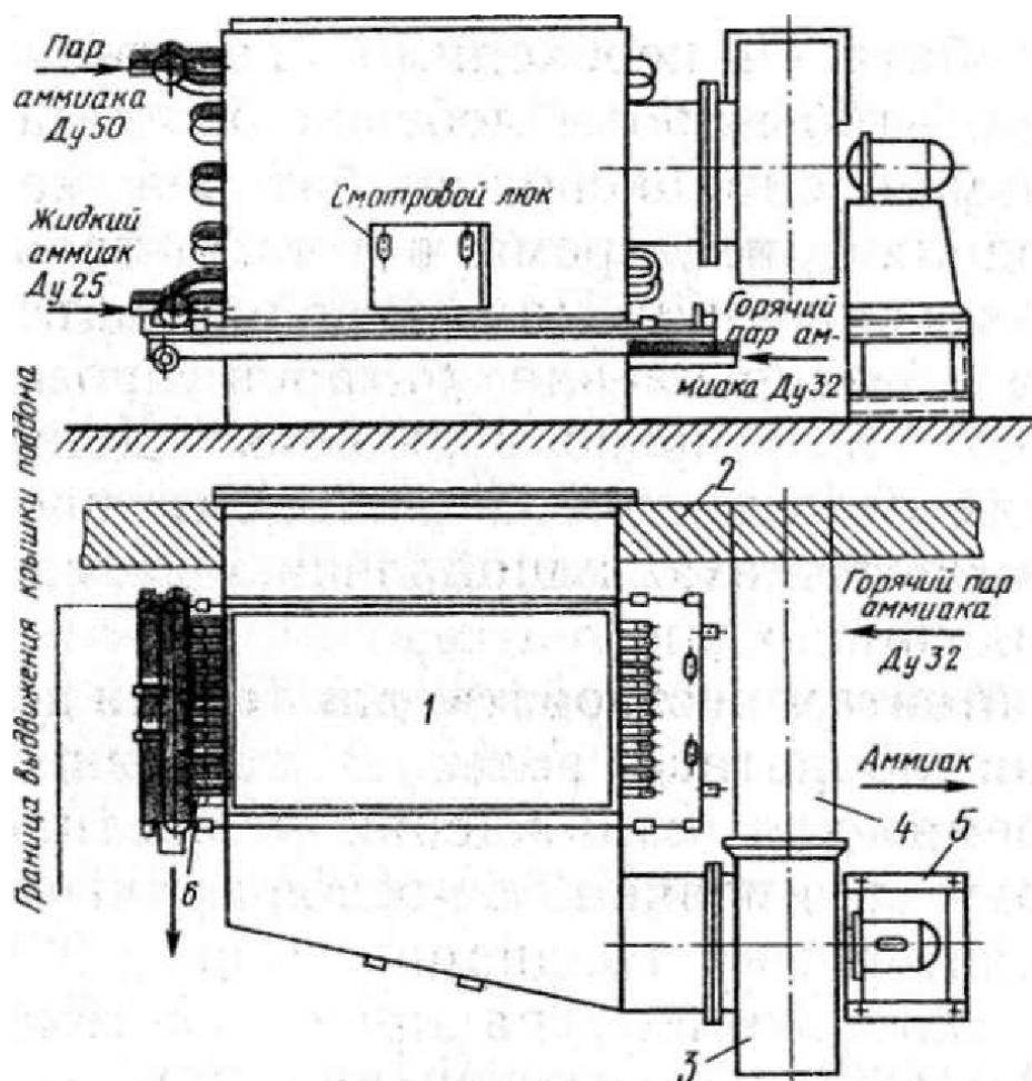
Рис. 5.4. Схема монтажа напольного воздухоохладителя:
