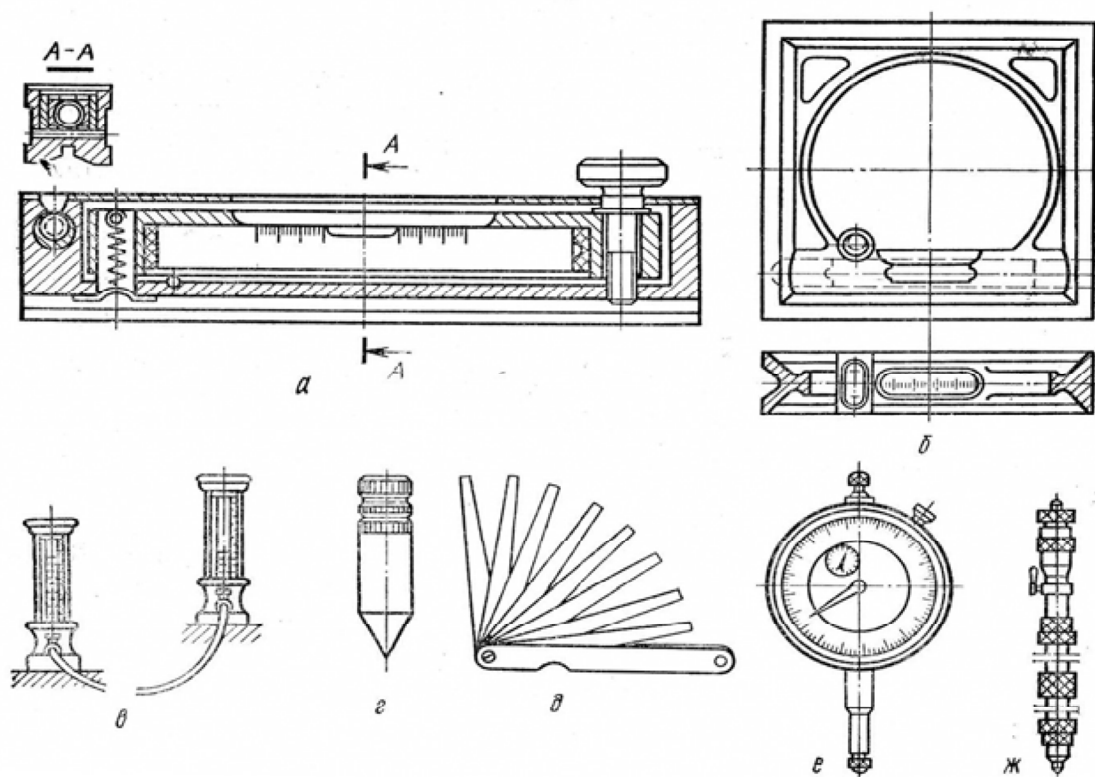
Рис. 2.6. Инструмент, применяемый при монтажных работах:
