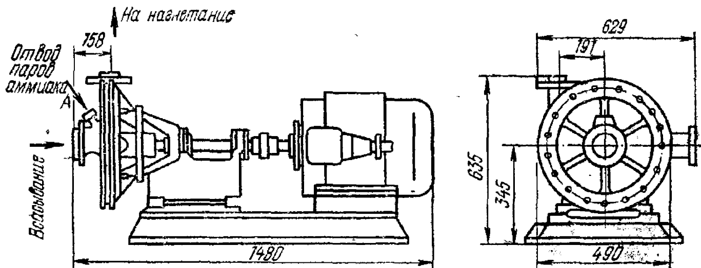
Рис. 6.3. Установочный чертеж аммиачных центробежных насосов марки ЗЦ-4 и ЗЦ-4А
