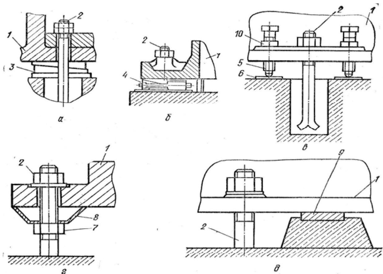
Рис. 2.7. Установка и выверка оборудования на подкладках и бесподкладочным методом: а - на клиновых подкладках; б - с помощью инвентарных винтовых домкратов; в - на установочных винтах; г - на установочных гайках; д - на жестких опорах; 1 - рама оборудования; 2 - фундаментный болт; 3 - клиновые подкладки; 4 - установочный домкрат; 5 - установочный винт; 6 - подкладная установочная пластина; 7 - установочная гайка; 8 - тарельчатая шайба; 9 - металлическая пластина с жесткой опорой; 10 - стопорная гайка.
