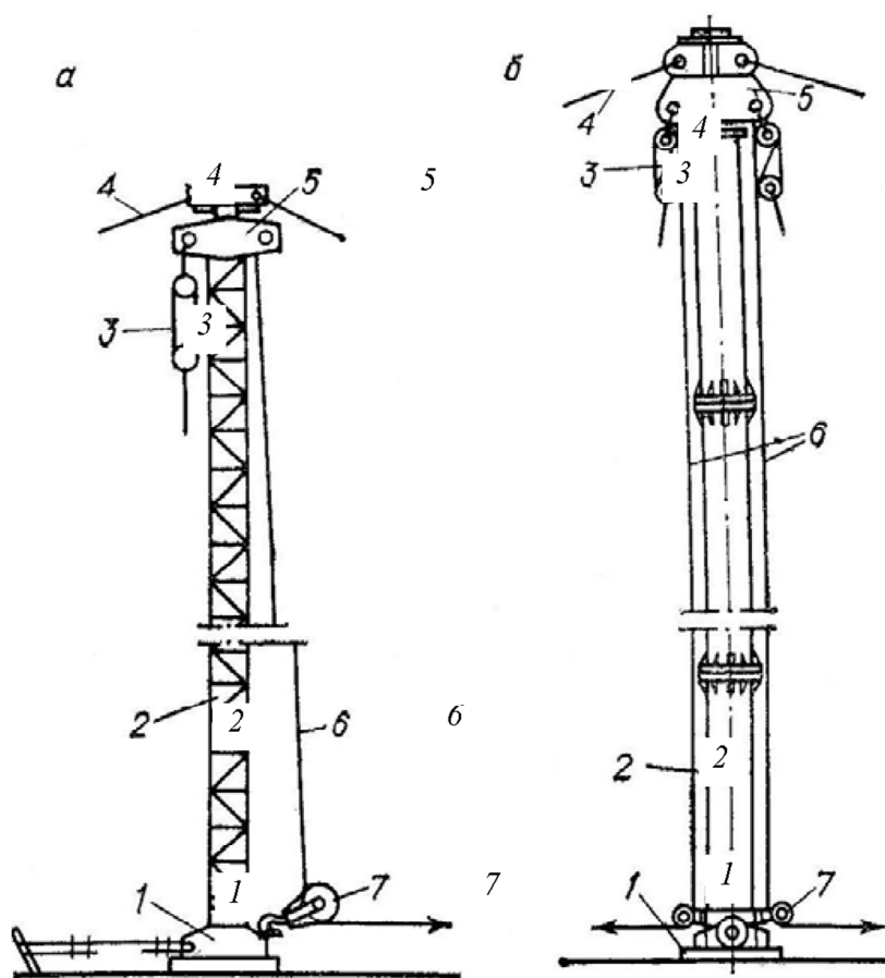
Рис. 1.1. Монтажные мачты: а - решетчатые; б - трубчатые; 1 - опорная пята; 2 - мачта; 3 - полиспаст; 4 - расчалка; 5 - оголовок; 6 - сбегающий канат; 7 - отводной блок
