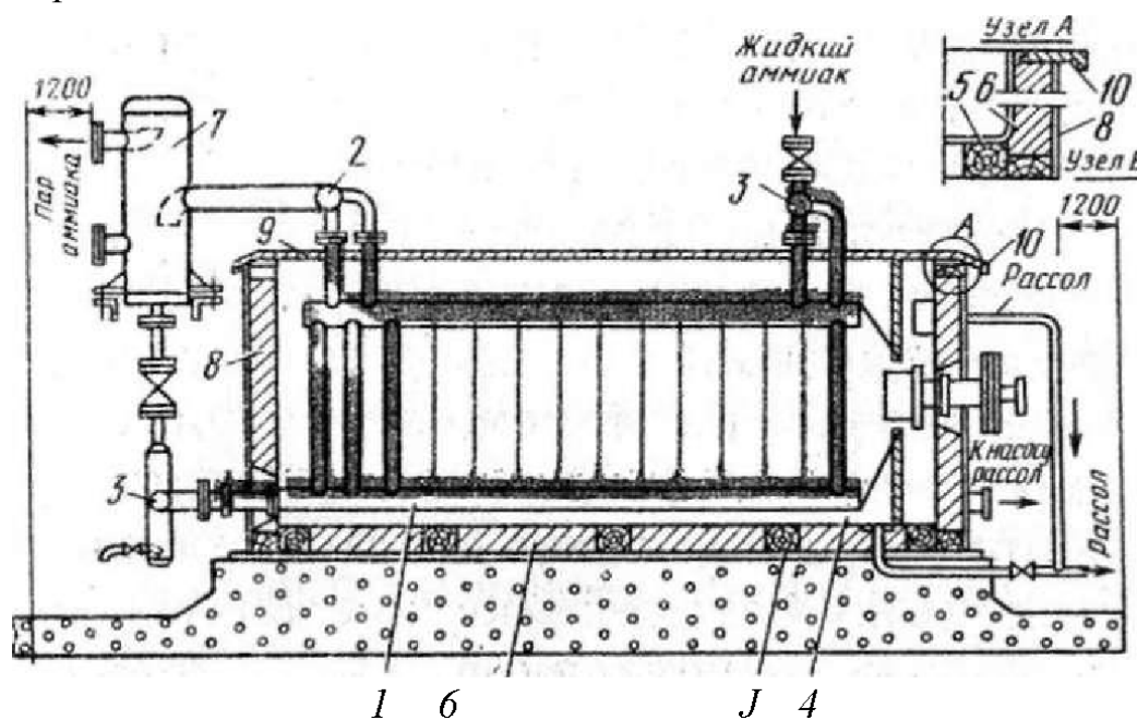
Рис. 5.3. Схема расположения рассольного панельного испарителя:
