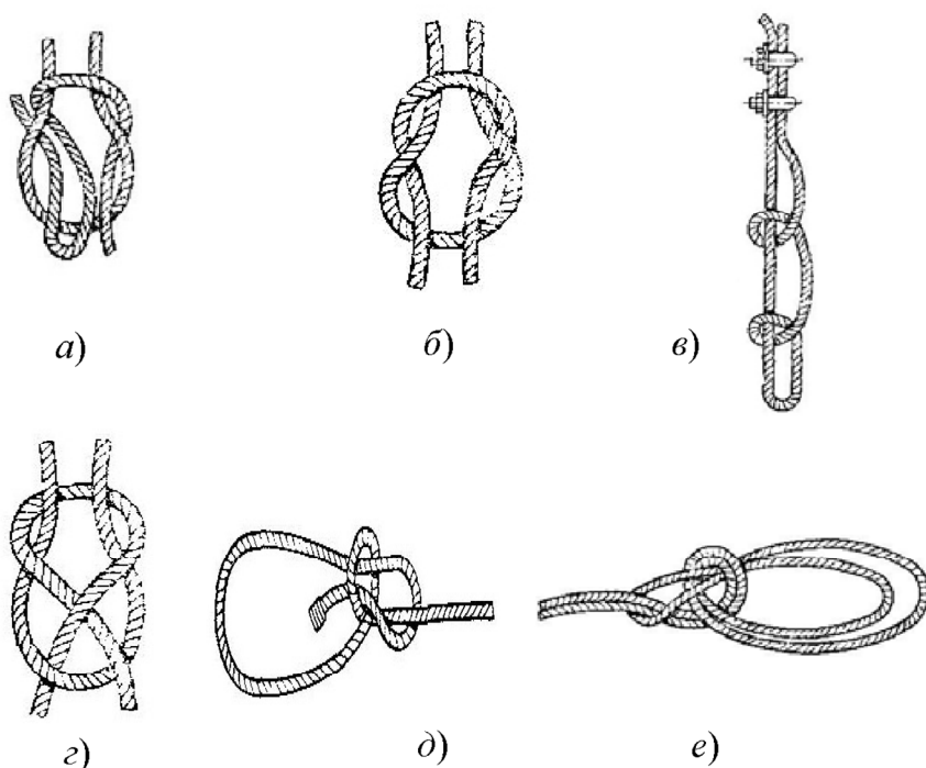
Рис.1.7. Способы вязки узлов: а - прямой; б - рифовый; в - штыковой для толстых пеньковых канатов; г - вязка в коуш или петлю; д - беседочный (морская петля); е - двойной беседочный
