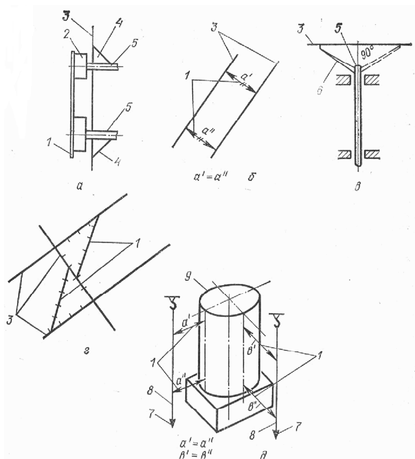
Рис. 2.9. Выверка параллельности и перпендикулярности осей, валов и аппаратов:
