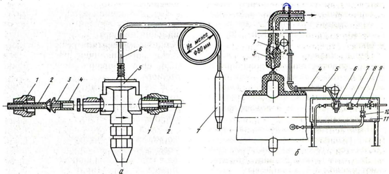
Рис. 8.7. Терморегулирующие вентили:
