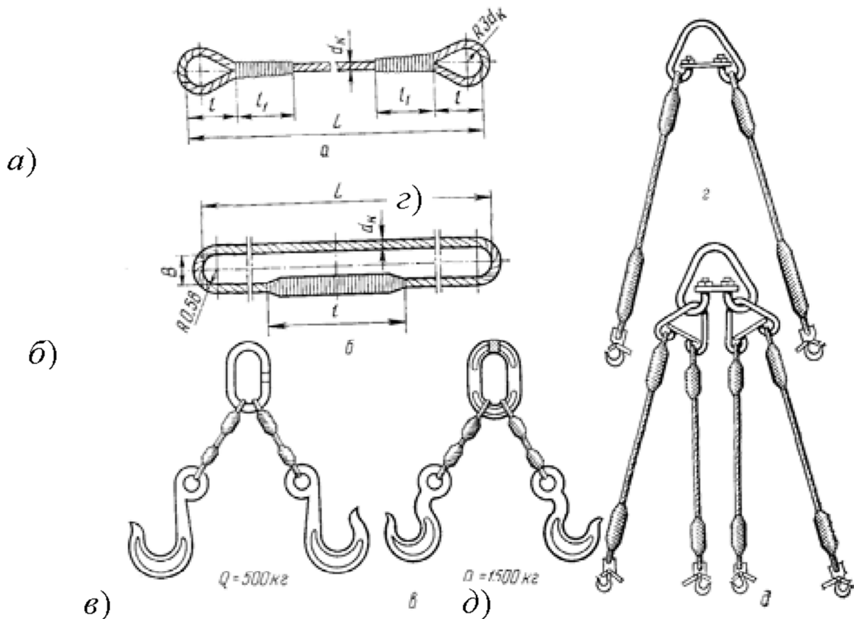
Рис. 1.8. Схемы строп:
