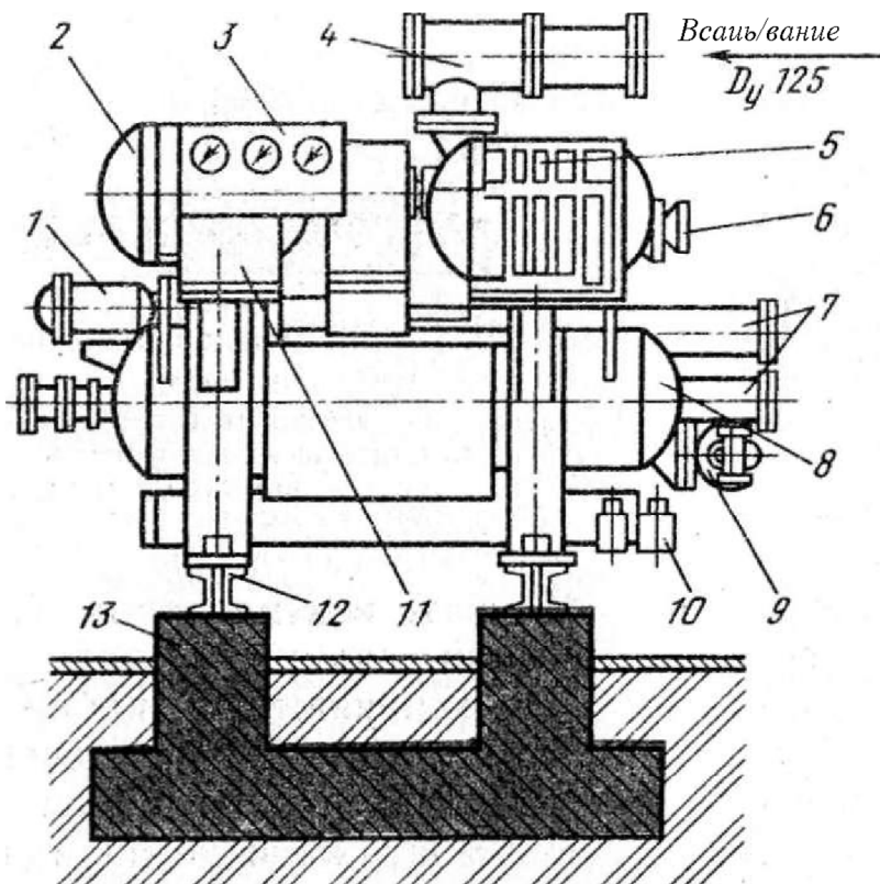
Рис. 4.5. Общий вид винтового компрессора на фундаменте:
