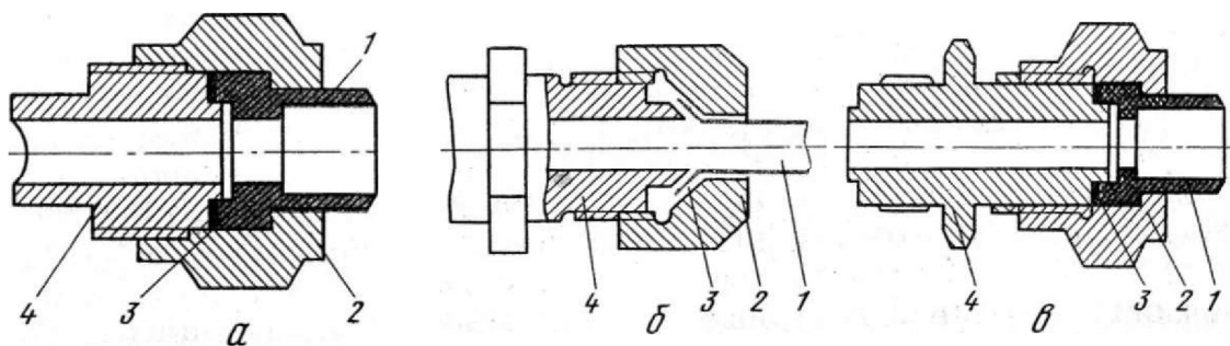
Рис. 7.2. Штуцерно-торцевые соединения:
