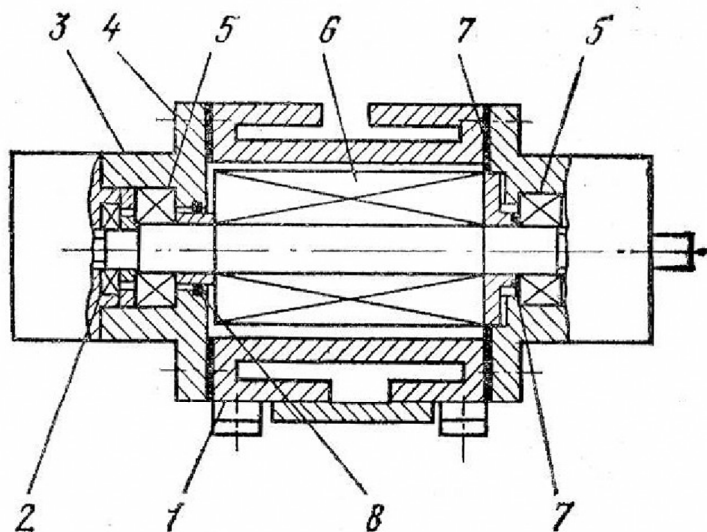
Рис. 4.4 . Ротационный компрессор: 1 - цилиндр; 2 - упорный подшипник; 3 - крышка; 4 - призонные болты или штифты; 5 - опорный подшипник; 6 - ротор с пластинами; 7 - прокладка; 8 - дистанционное кольцо.
