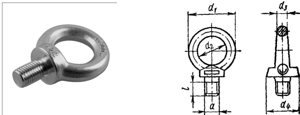
Рис. 1.11. Рым-болты
