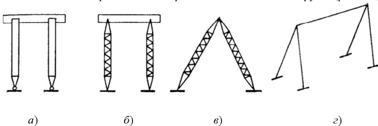
Рис. 1.2. Схема порталов:
