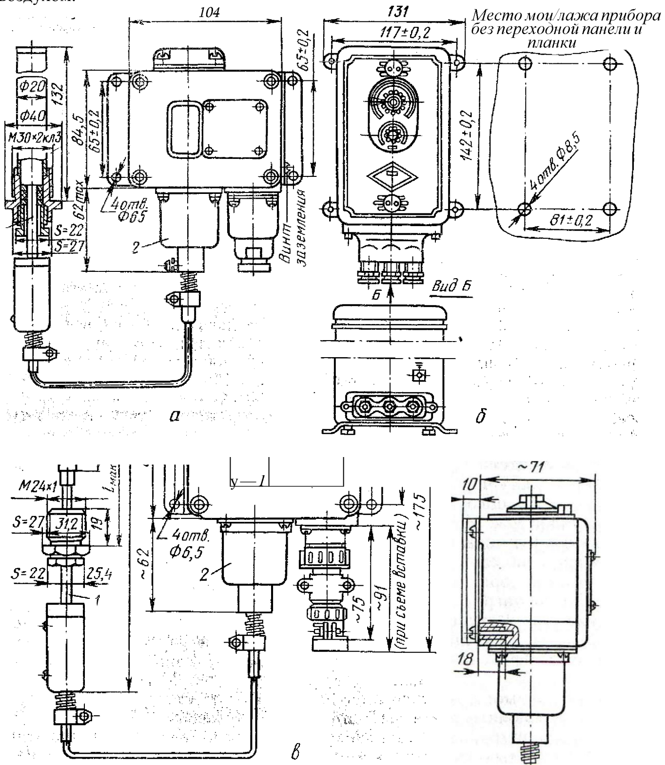
Рис. 8.1. Реле температуры:
