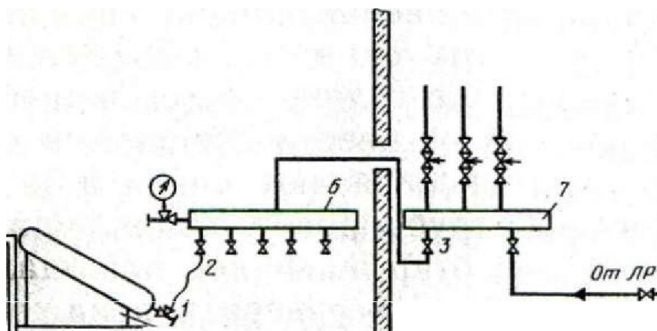
Рис. 9.3. Схема заправки системы аммиаком из баллонов:
