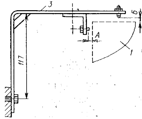
Рис. 4.2. Приспособление для проверки соосности валов с эластичной муфтой:
