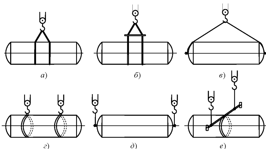
Рис. 1.21. Схемы строповки горизонтальных аппаратов:
