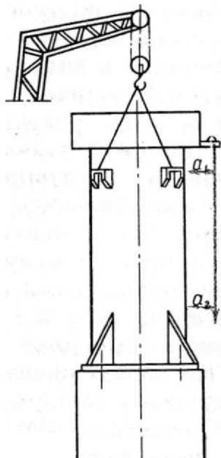
Рис. 5.2. Схема проверки положения вертикального конденсатора
