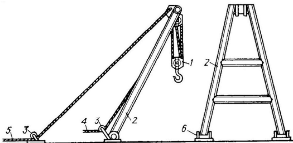
Рис. 1.3. Схема шевра:
