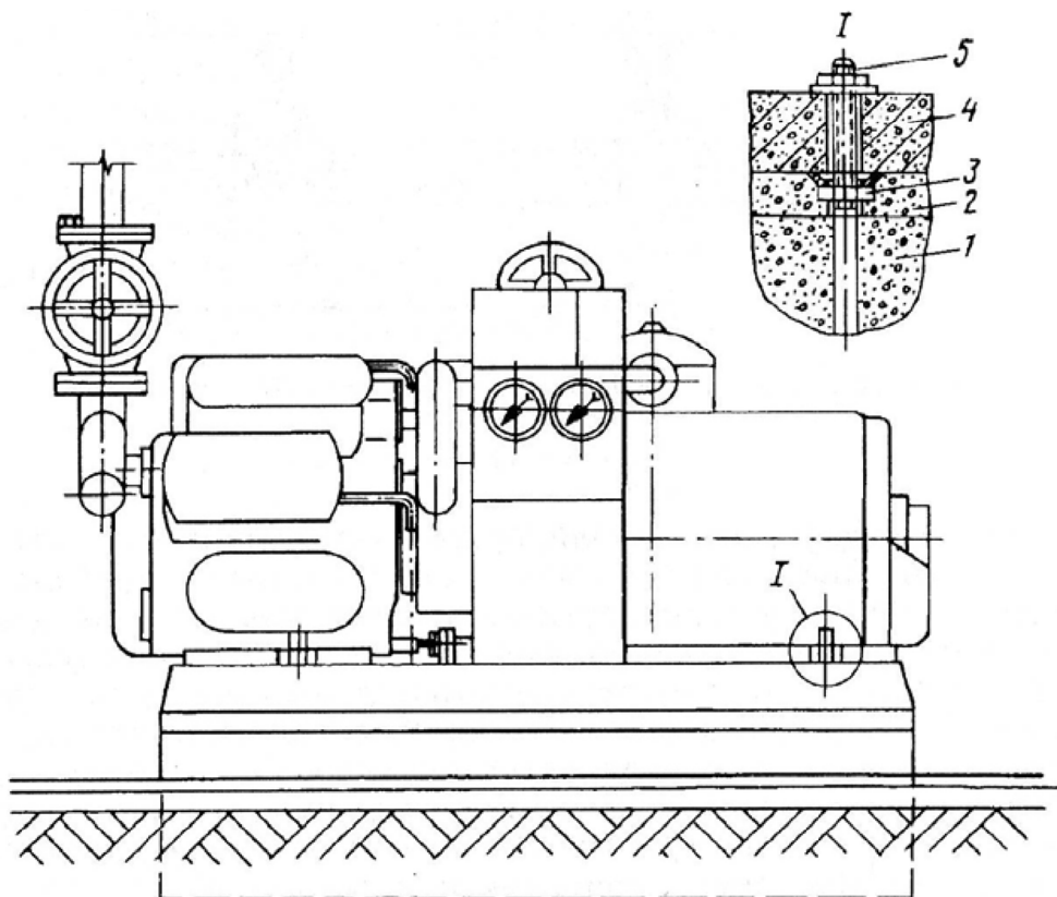
Рис. 4.3. Размещение поршневого компрессорного агрегата на фундаменте: 1 - бетонный фундамент; 2 - бетонная подливка; 3 - выверочная гайка с конической шайбой; 4 - железобетонная рама; 5 - фундаментный болт.
