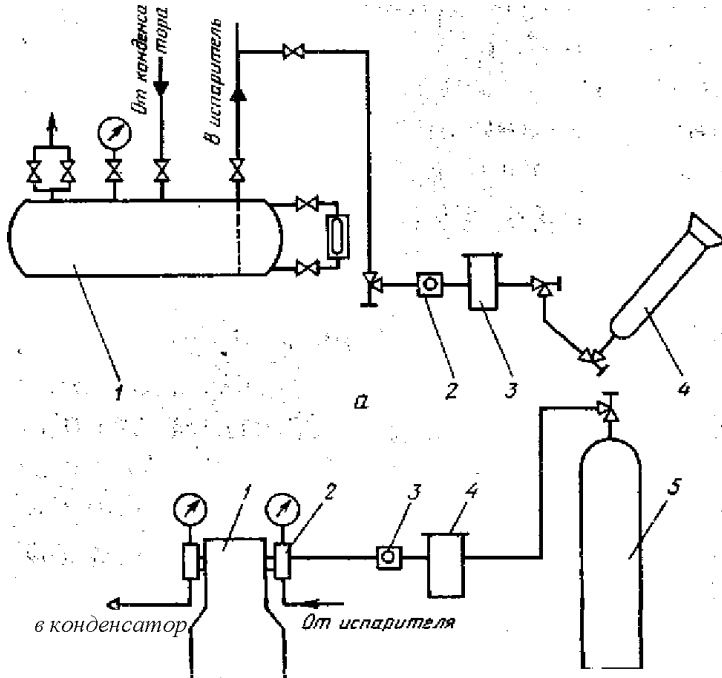
Рис. 9.4. Схема заправки хладоном машин:
