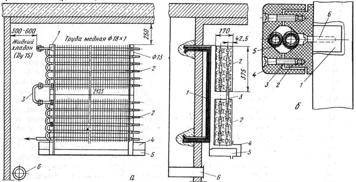
Рис. 3.2. Схема монтажа хладоновых батарей и трубопроводов:
