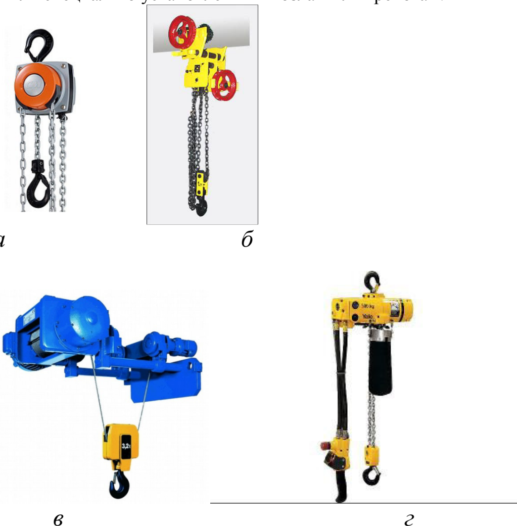
Рис. 1.14. Тали
