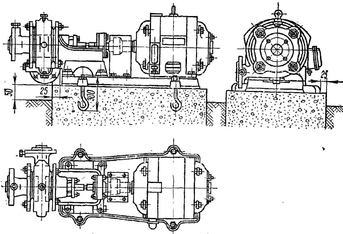
Рис. 6.4. Установочный чертеж центробежного насоса типа К
