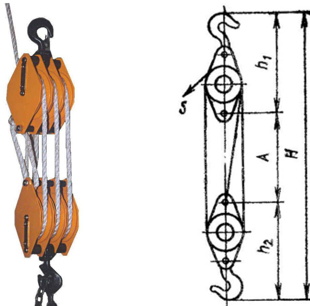
Рис. 1.12. Полиспасть
