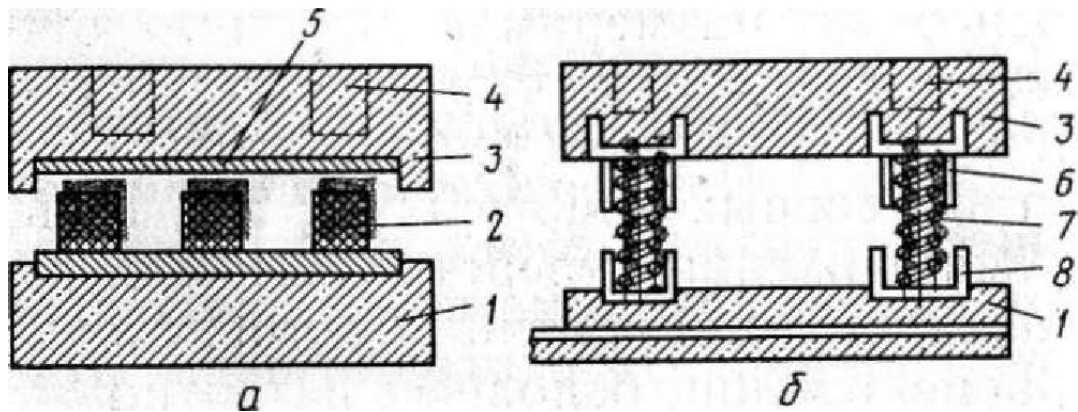
Рис. 2.2. Виброизоляционные фундаменты на резиновых (а) и пружинных амортизаторах (б): 1 — железобетонные плиты; 2 — резиновые пластины; 4 — колодцы для болтов; 5 — антисептированные доски; 6 — верхний стакан; 7 — пружина; 8 — нижний стакан
