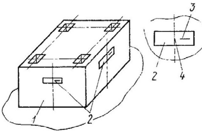
Рис. 2.4. Схема планки для нанесения на фундаментах осей и высотных отметок: 1 - фундамент; 2 - планка; 3 - высотная отметка; 4 - осевая отметка
