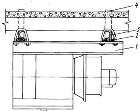
Рис. 5.6. Крепление подвешеного воздухоохладителя к бетонным несущим конструкциям:
