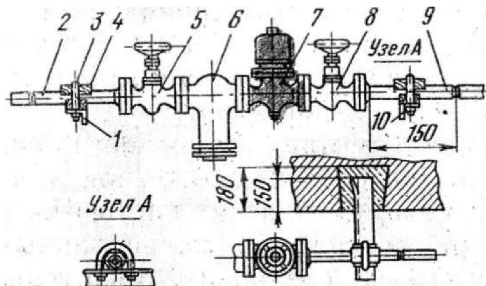
Рис. 8.8. Узел монтажа СВМ соленоидного вентиля трубопровода:
