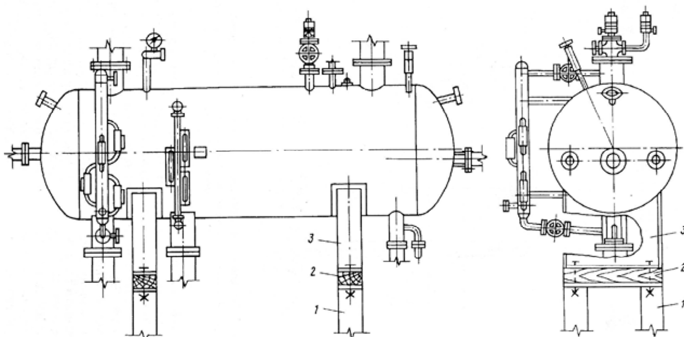
Рис. 6.2. Размещение на фундаменте циркуляционного ресивера:
