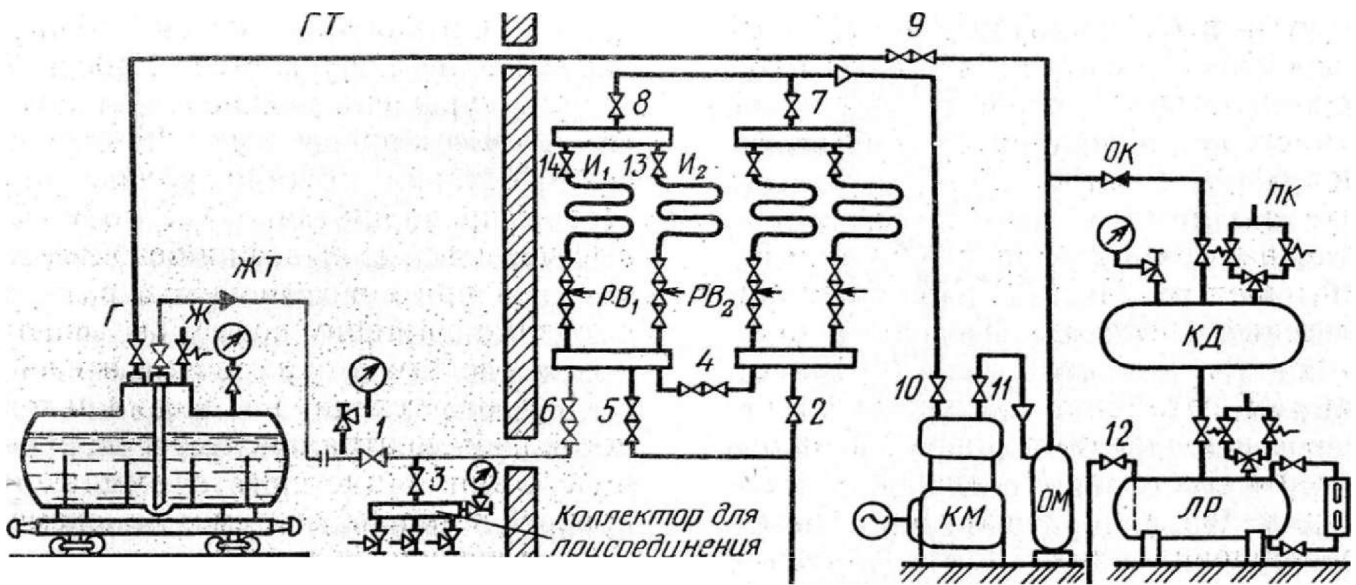
Рис. 9.1. Схема слива аммиака из цистерны:
