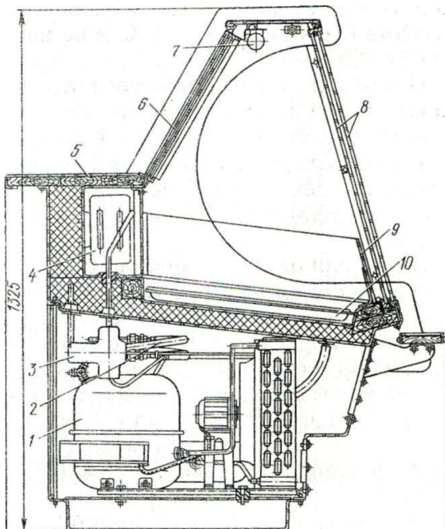
Рис. 3.1. Разрез прилавка-витрины «Пингвин-В»:
