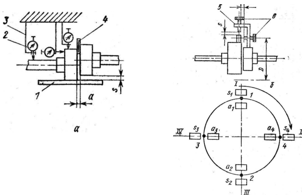
Рис.2.8. Схемы центровки валов:
