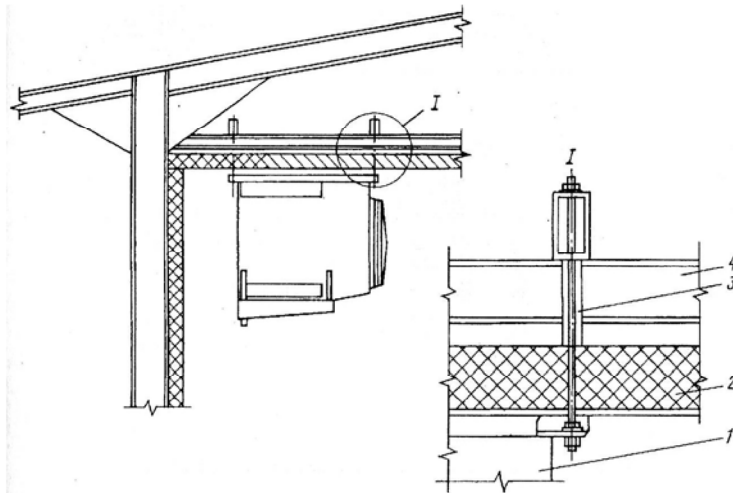
Рис. 5.7. Крепление подвешеного воздухоохладителя к металлическим несущим конструкциям:
