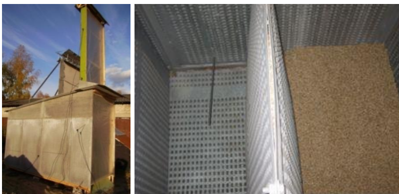
Рисунок 10 – Общий вид зернохранилища со встроенной гелиосистемой
