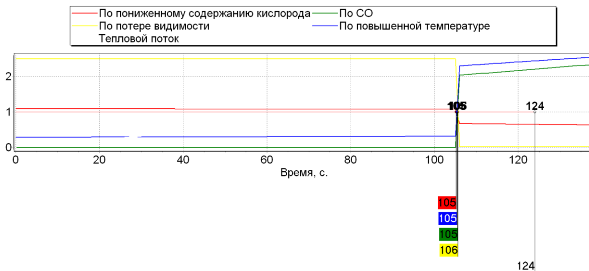
Рисунок 4 - Результаты расчетов для помещения (рт_02)
