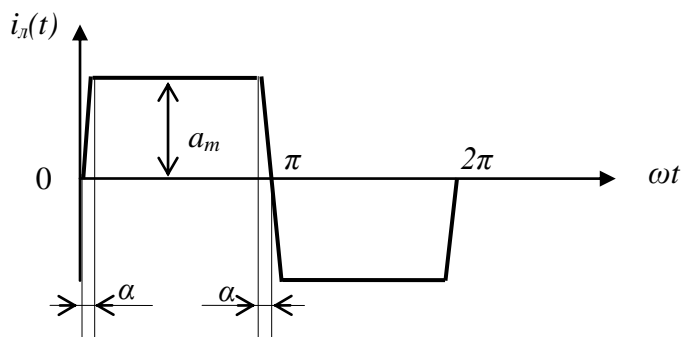
Рисунок 3. Параметры аппроксимированной трапецевидной кривой тока i_n(t) : a_m – амплитудное значение кривой i_n(t) ; \alpha = \pi/12
