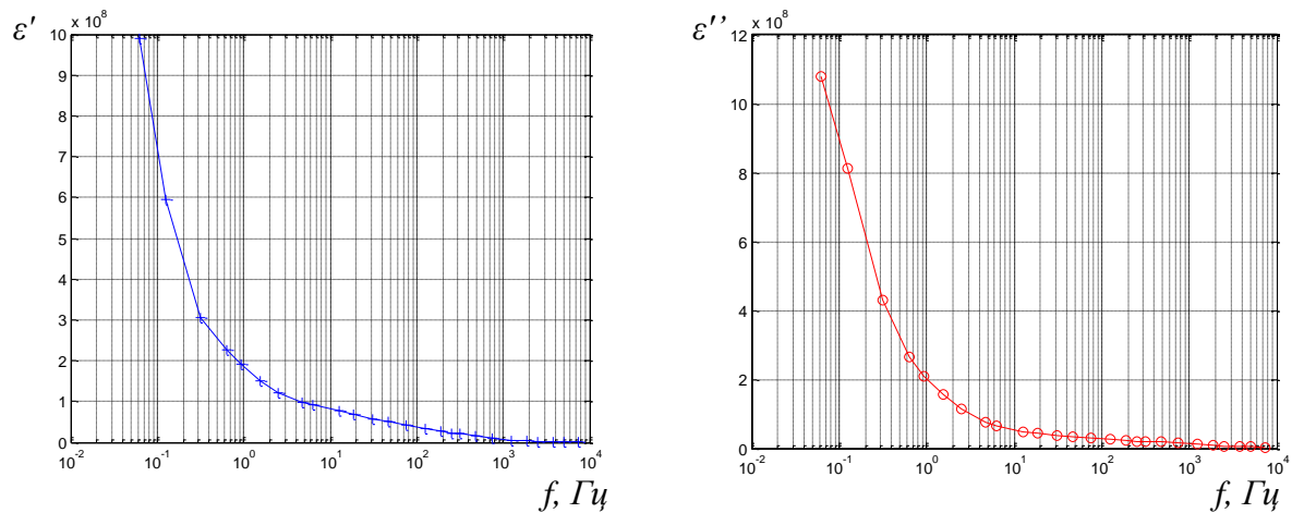
Рисунок 6 – Частотные зависимости КДП (серая лесная почва, горизонт В 1 )
