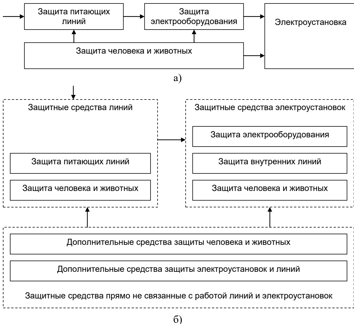
Рисунок 1. Система защит производственного помещения (а) и обобщенная структура защит производственного помещения (б)
