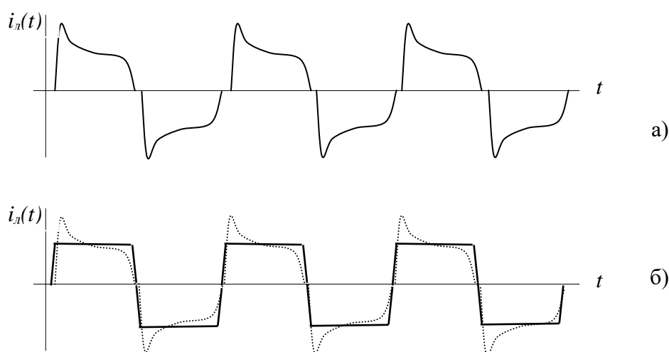
Рисунок 2. Аппроксимация кривой тока i_l(t) а) через лампу с индуктивным балластом трапециевидной кривой б)
