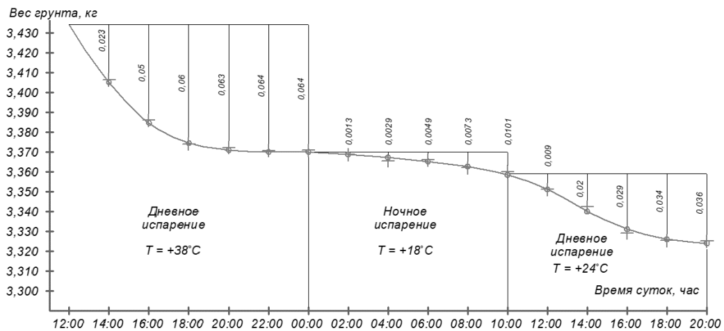
Рис. 4. Обобщённый график испарения за 1,5 суток в полевых условиях
