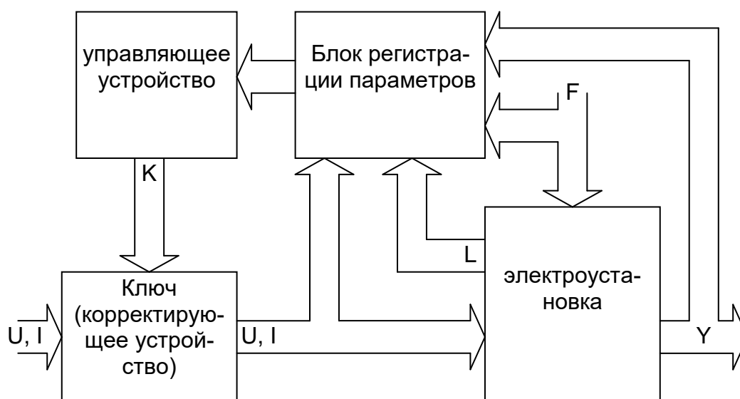
Рисунок 4. Типовая структура комбинированного защитного аппарата с общим ключом
