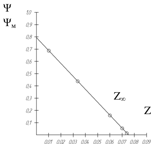
Рис. 2. Зависимость \Psi_M = f(Z) для дневного периода
