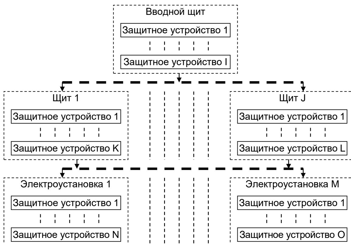
Рисунок 2. Структура защит производственного помещения
