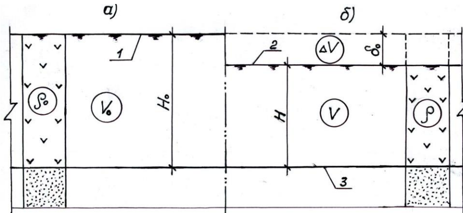
Рис. 1. Графическая иллюстрация изменения торфяника при его осушении
