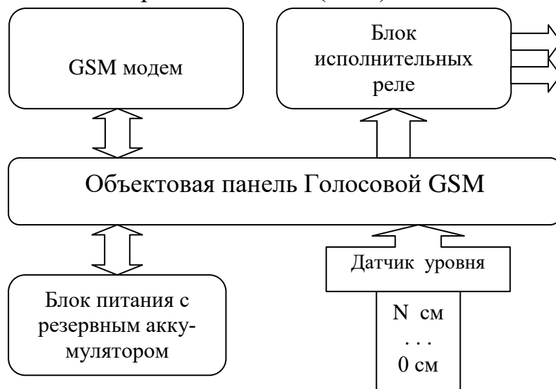
Рис. 1. Структурная схема АСК (автоматизированная система контроля).
