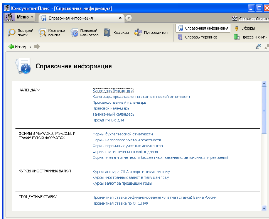
Рис. 20. Справочная информация
