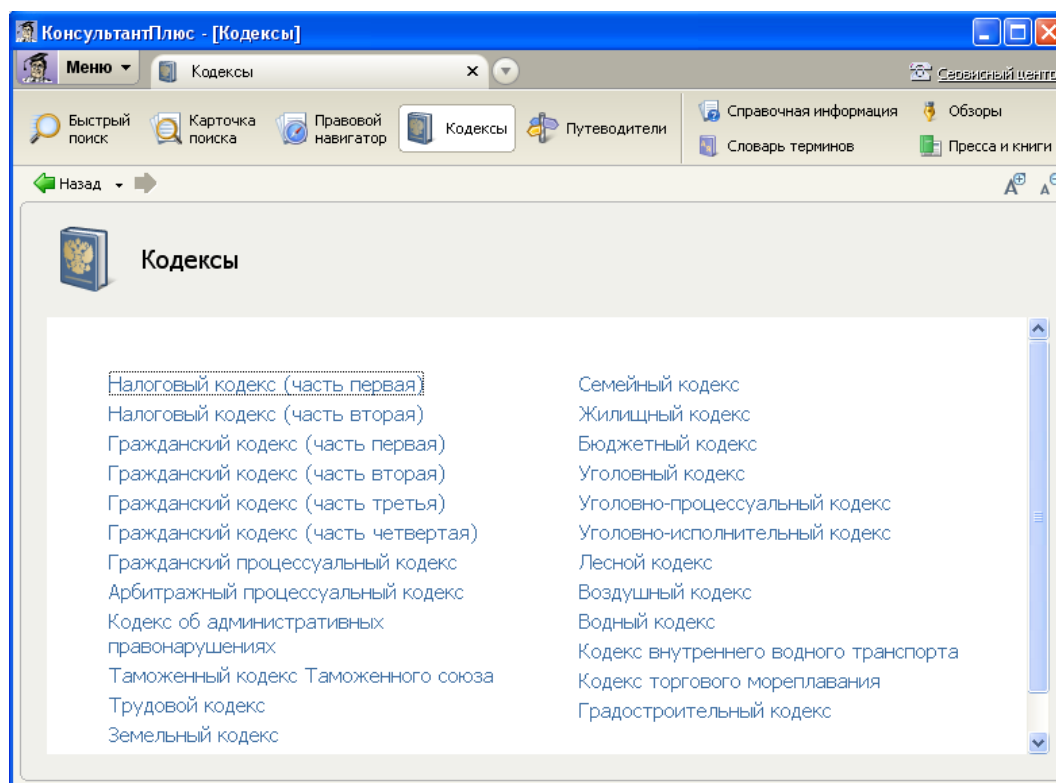
Рис. 17. Окно Кодексы
