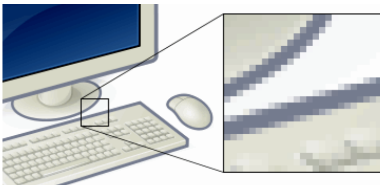
Рис. 2. Растровое изображение
