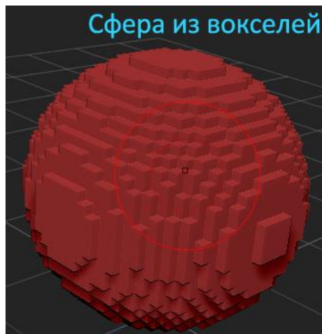
Рис. 6. Воксельная графика
