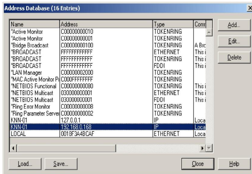
Рис. 5.7. Окно работы с базой данных адресов
