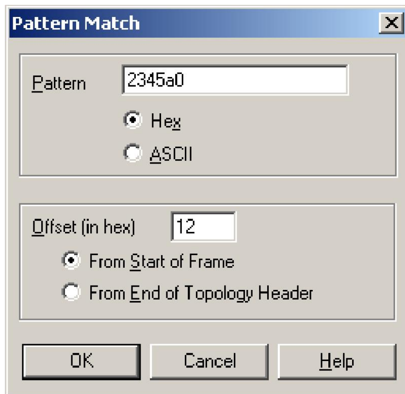
Рис. 5.11. Окно задания шаблона фильтрации при захвате. Единожды созданные критерии могут быть сохранены в отдельном файле и затем многократно использоваться.
