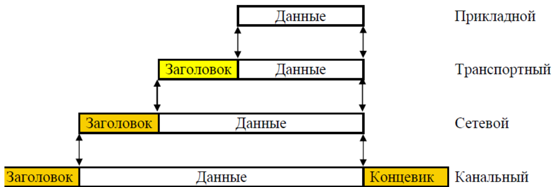
Рис. 5.1. Принцип инкапсуляции в стеке протоколов
