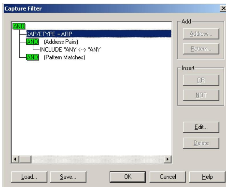
Рис. 5.8. Окно выбора критериев фильтрации при захвате
