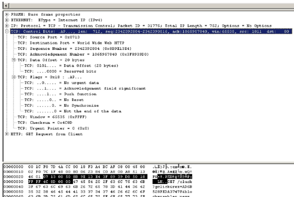
Рис. 5.13. Развернутое отображение полей протокола TCP анализируемого кадра
