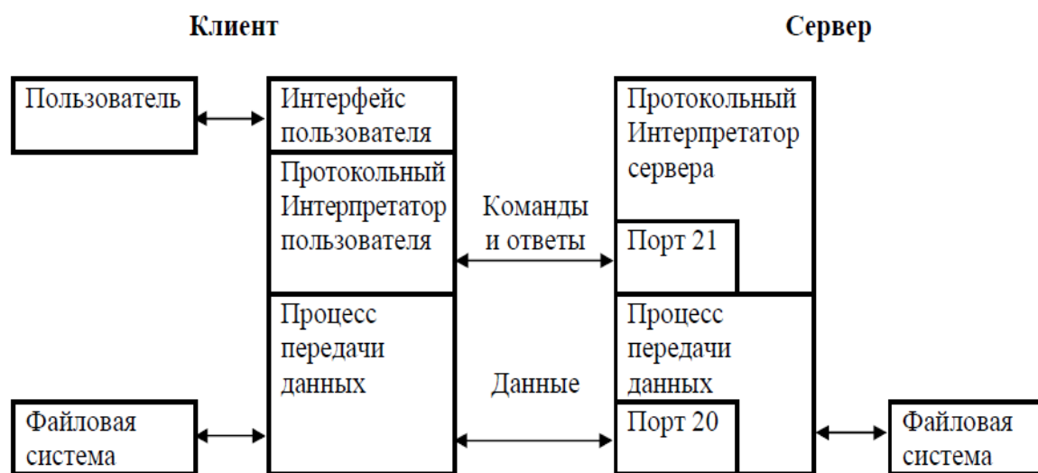
Рис. 6.1. Схема взаимодействия клиента и сервера FTP
