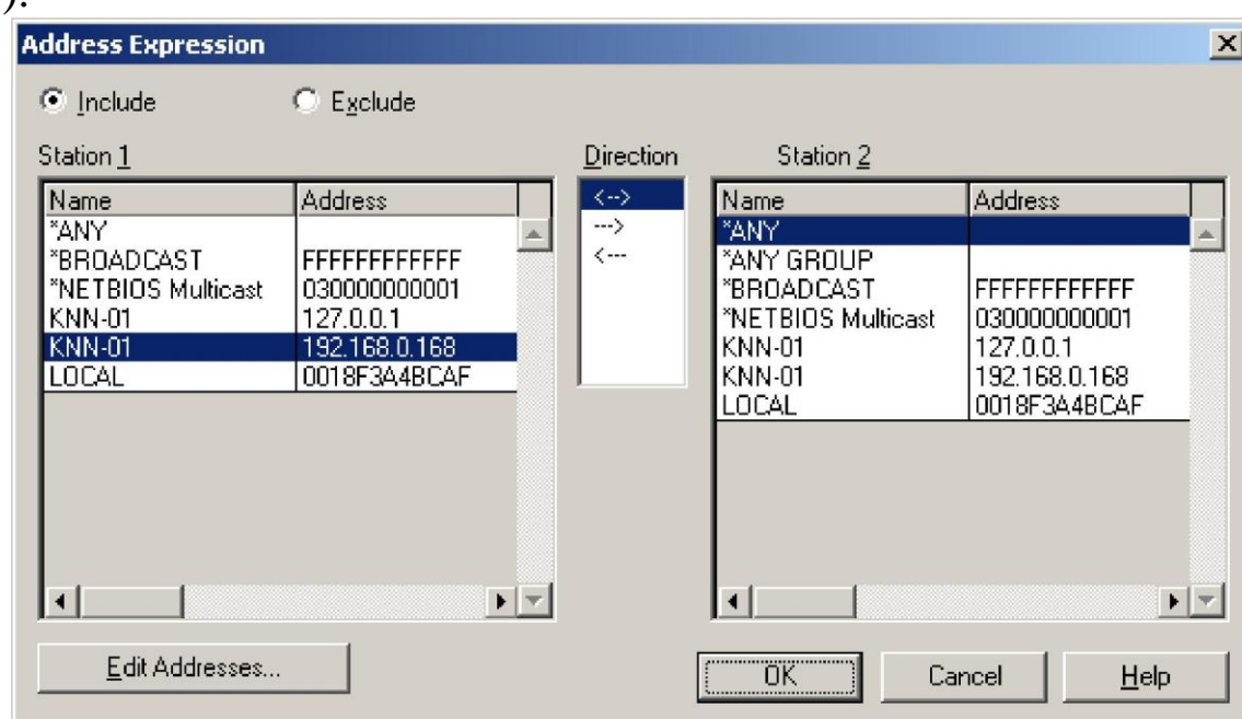
Рис. 5.10. Окно задания адресных пар фильтрации при захвате
