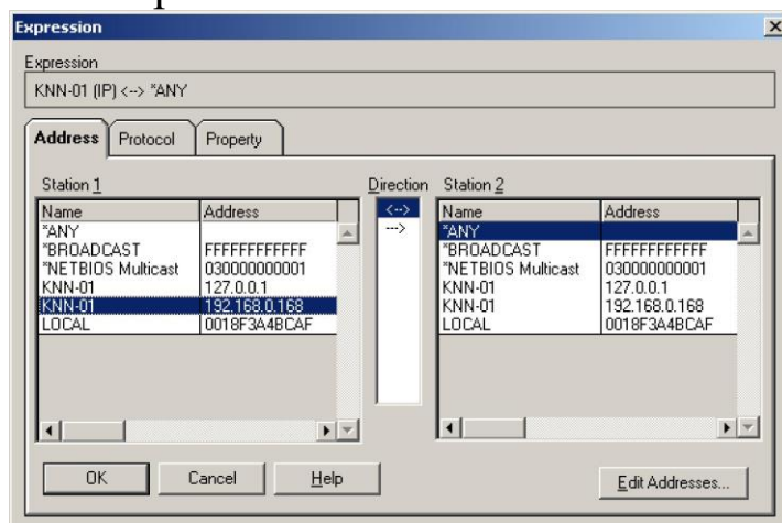
Рис. 5.15 Диалоговое окно для задания адресов, протоколов или свойств протоколов
