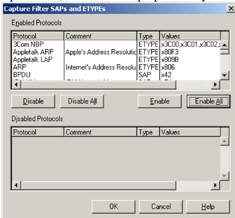
Рис. 5.9. Окно выбора протокола фильтрации при захвате
