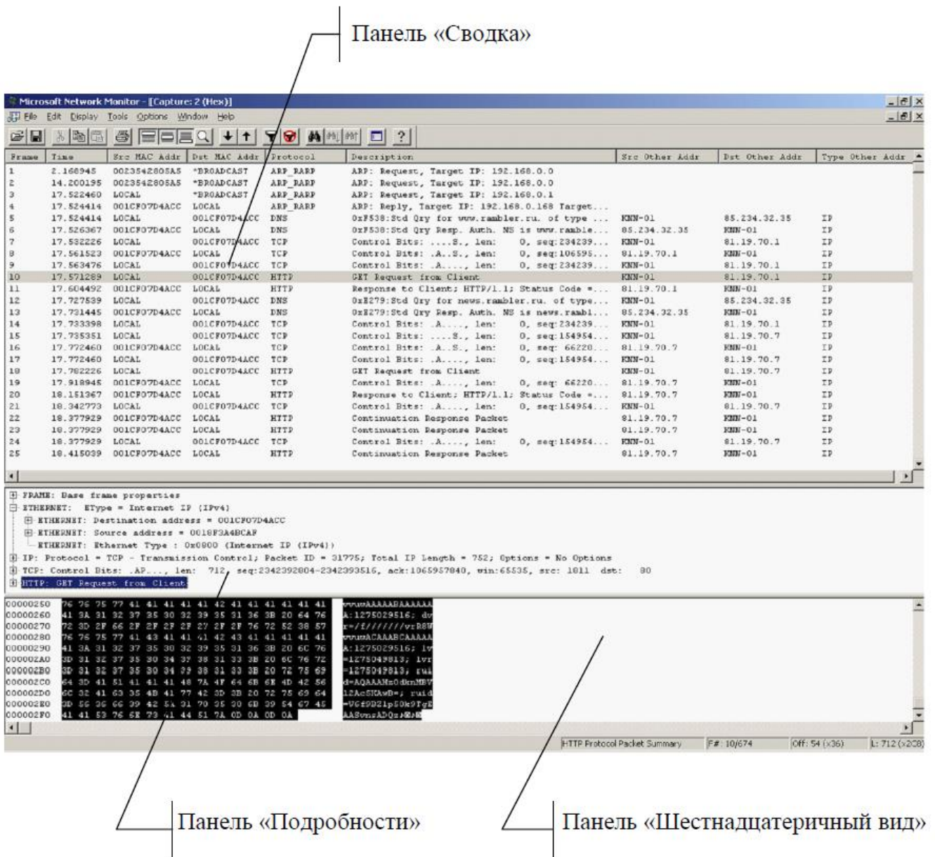
Рис. 5.12. Окно записи данных
