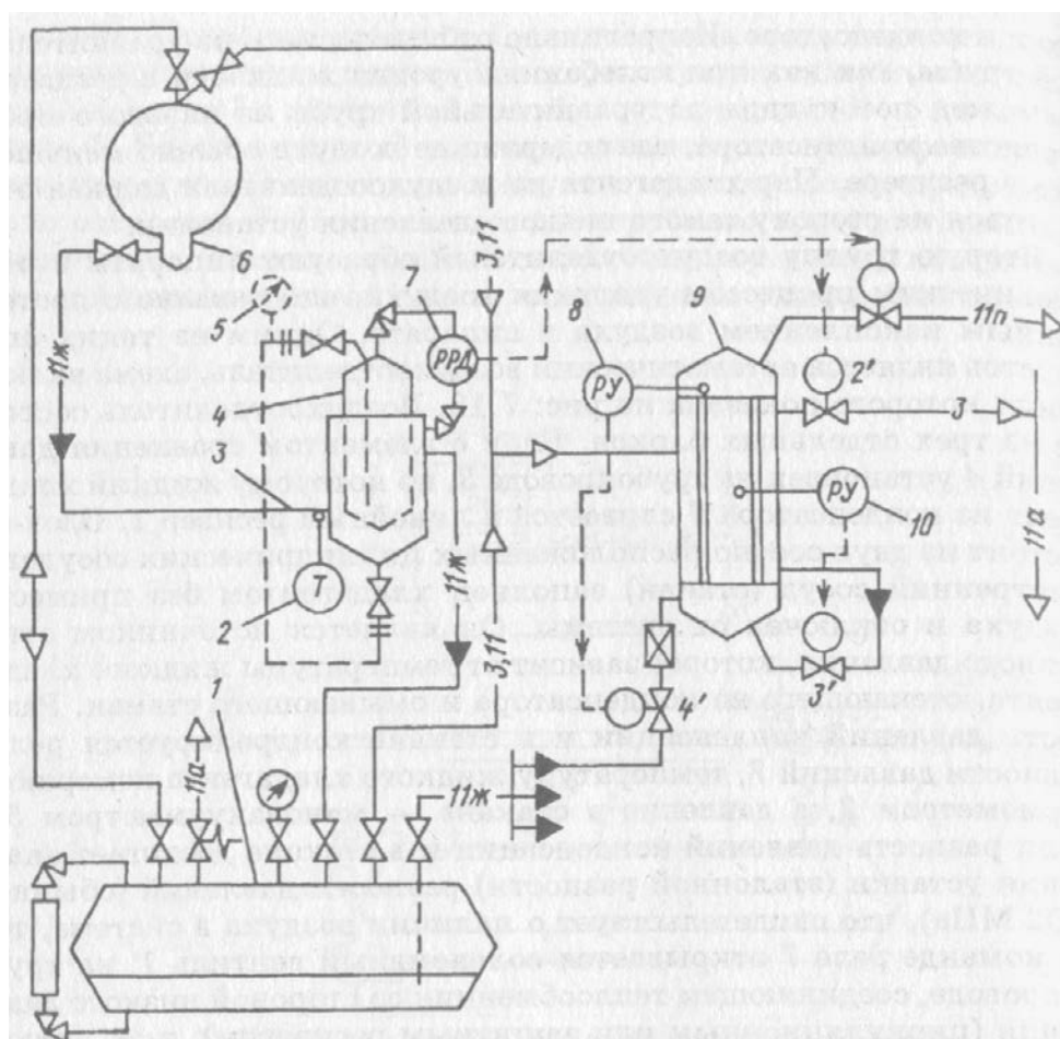
Рис. 2.5. Автоматически воздухоотделитель:
