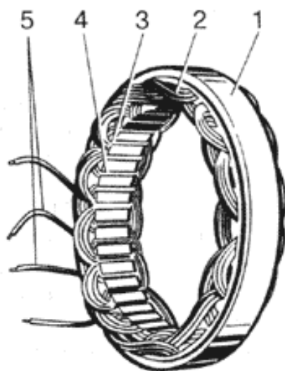
Рисунок 5 – Статор генератора:
