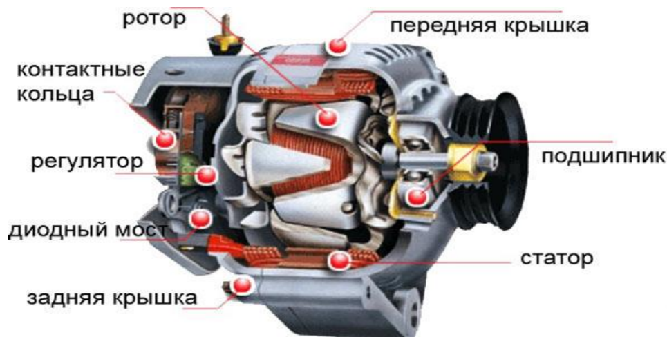
Рисунок 3 – Генератор
