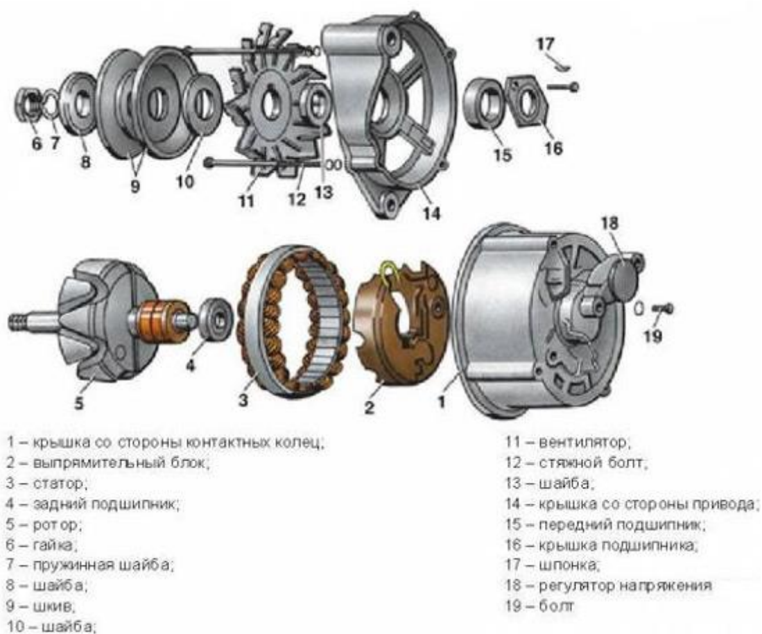
Рисунок 4 – Устройство генератора
