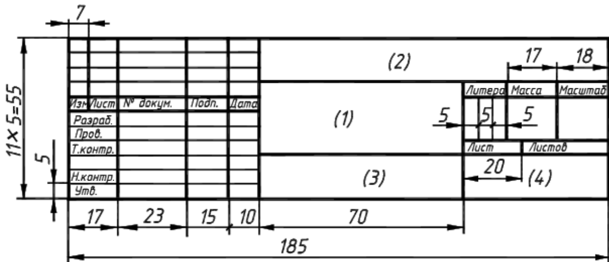
Рисунок 2 - Основная надпись чертежа
