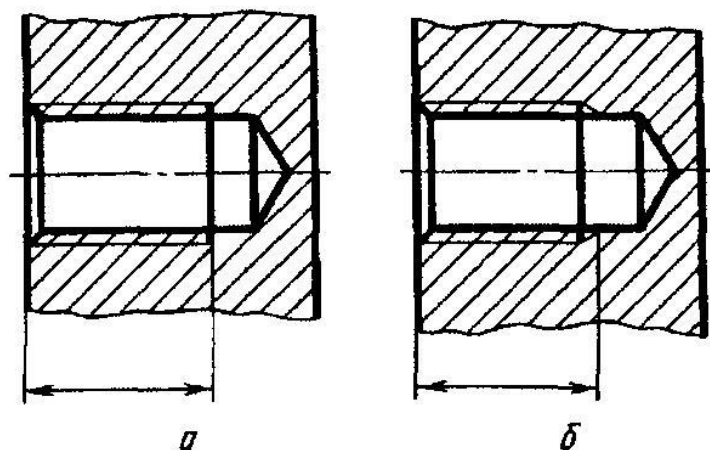
а – без сбега; б – со сбегом.
