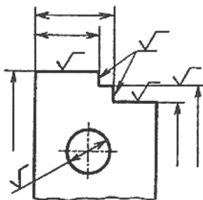
Рисунок 13 – Пример обозначения шероховатости на чертеже
