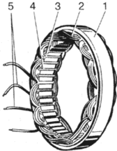
Рисунок 5 - Статор генератора:
