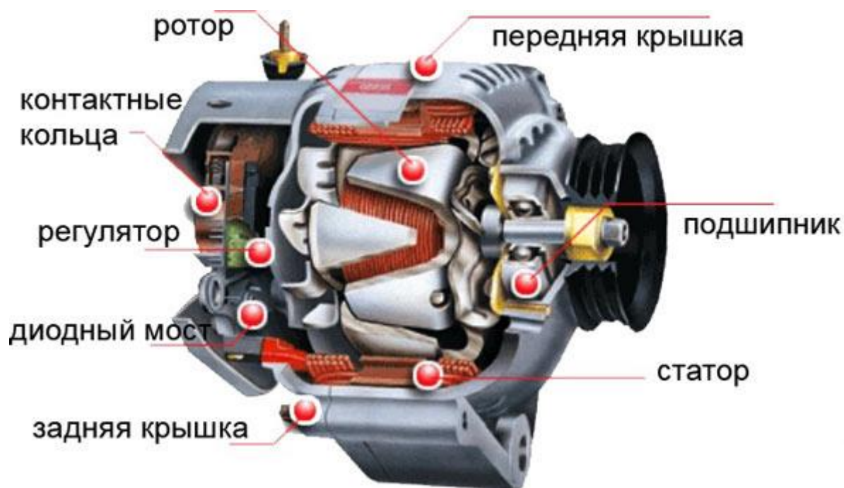
Рисунок 3 - Генератор
