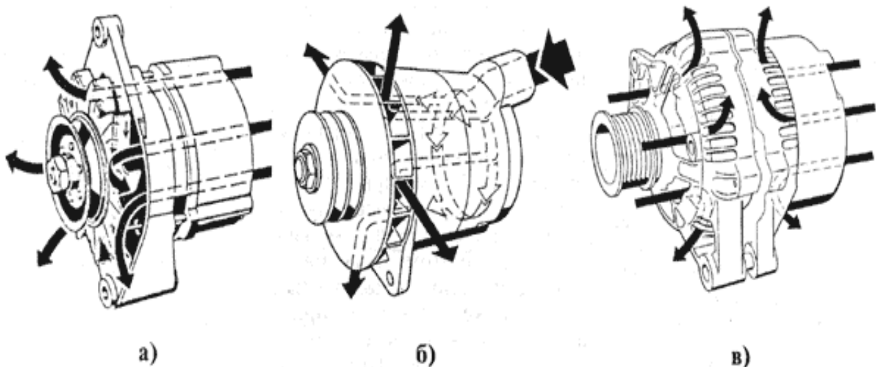
Рисунок 7 - Система охлаждения генераторов:
