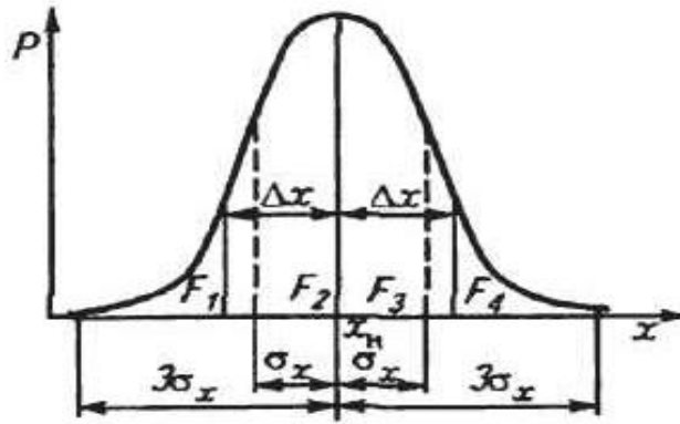
Рис. 9.1. График нормального распределения
