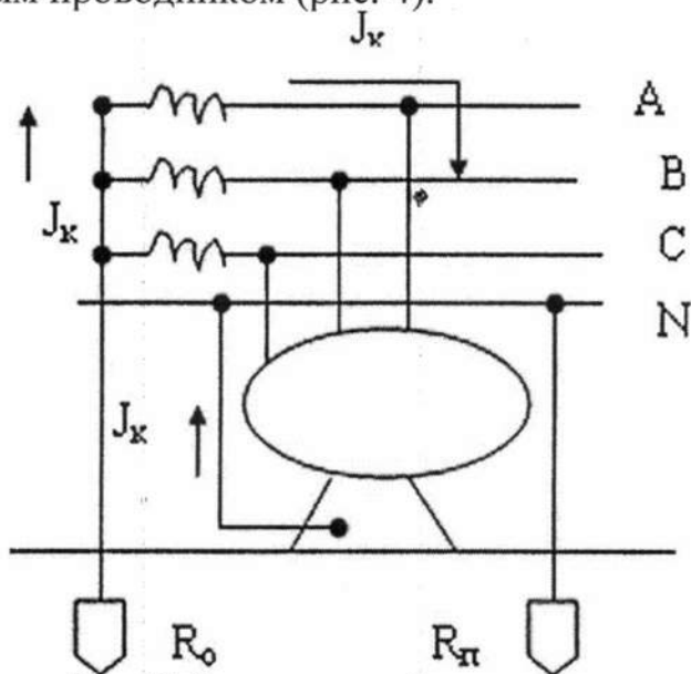
Рис. 9. Зануление оборудования
