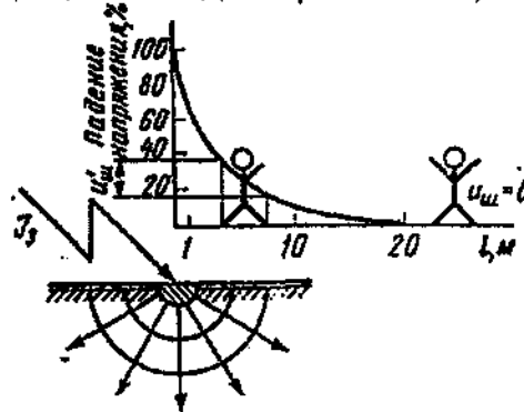
Рис. 4. Распределение потенциала на поверхности земли при прикосновении человека, не изолированного от земли, к нетоковедущим металлическим частям (корпусам) электроустановок, оказавшихся под напряжением из-за замыкания на корпусе;
