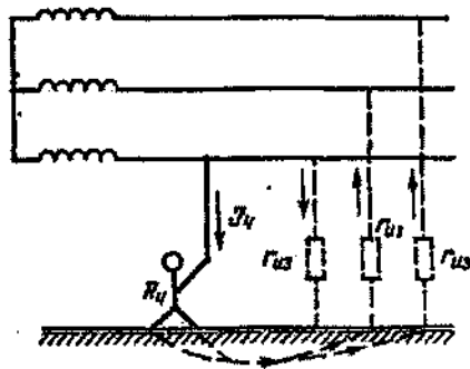
Рис. 2. Однофазное включение в сеть с изолированной нейтралью
