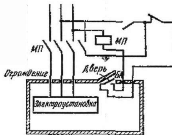
Рис. 7. Схема электрической блокировки
