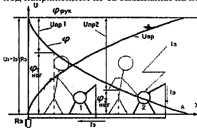
Рис. 5. Напряжение прикосновения
