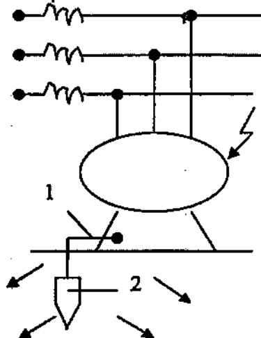
Рис. 8. Схема защитного заземления
