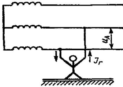
Рис. 3. Двухфазное включение человека в трехфазную сеть
