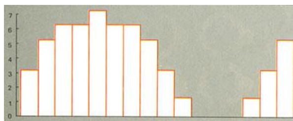
Рис. 2. Дискретный сигнал
