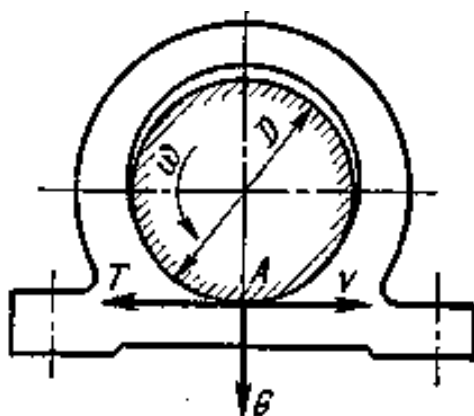
Рис. 3.4 - Схема сил, возникающих в подшипнике скольжения при вращении вала
