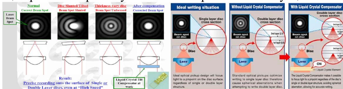
Рис. 40. Принцип работы Liquid Crystal Element
