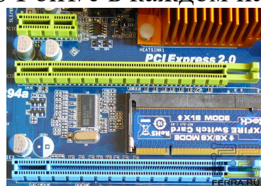
Рис. 23. Слоты PCI-E. Длинные для видеокарт короткий – для плат рас-
