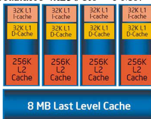
Рис. 9. Уровни кэш – памяти процессора Core i7-3770 K
