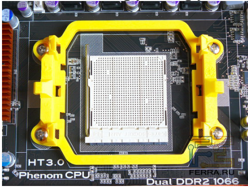
Рис. 16. Разъем Socket AM2/AM2+/AM3 для процессоров AMD Athlon/Phenom/Phenom II
