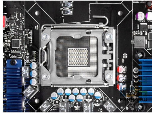
Рис. 17. Разъем Socket LGA1366 для процессоров Intel Core i7
