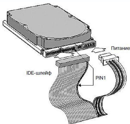
Рис. 65. Подключение IDE-устройства
