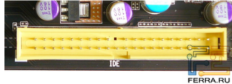
Рис. 26. Разъем IDE
