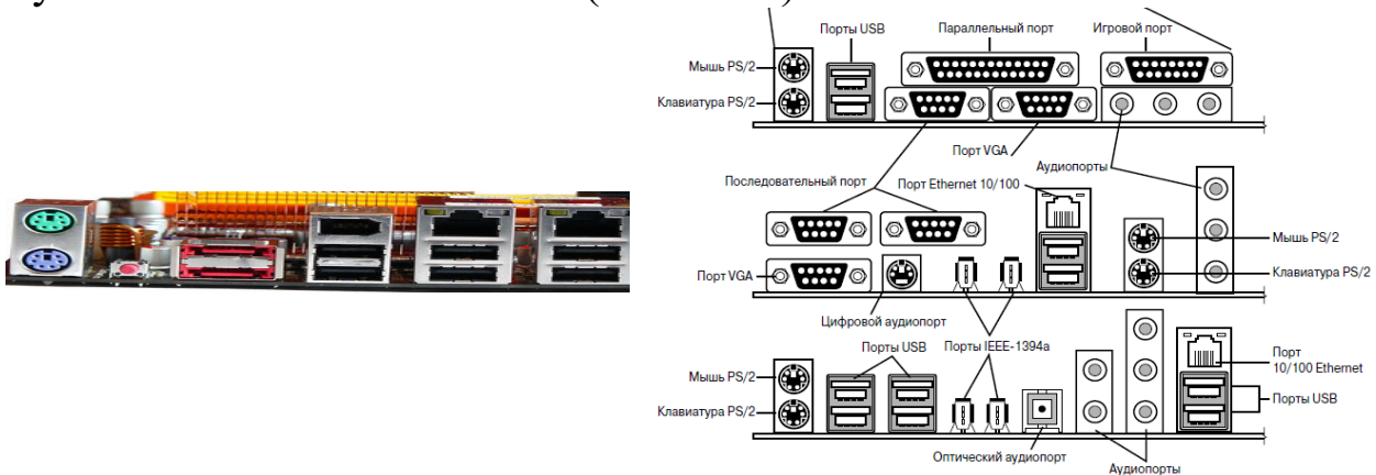
Рис. 33. Задняя панель материнской платы
