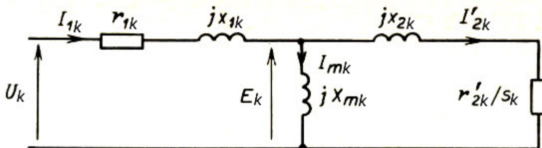
Рис. 1. Однофазная схема замещения асинхронного двигателя на частоте k – той гармоники
