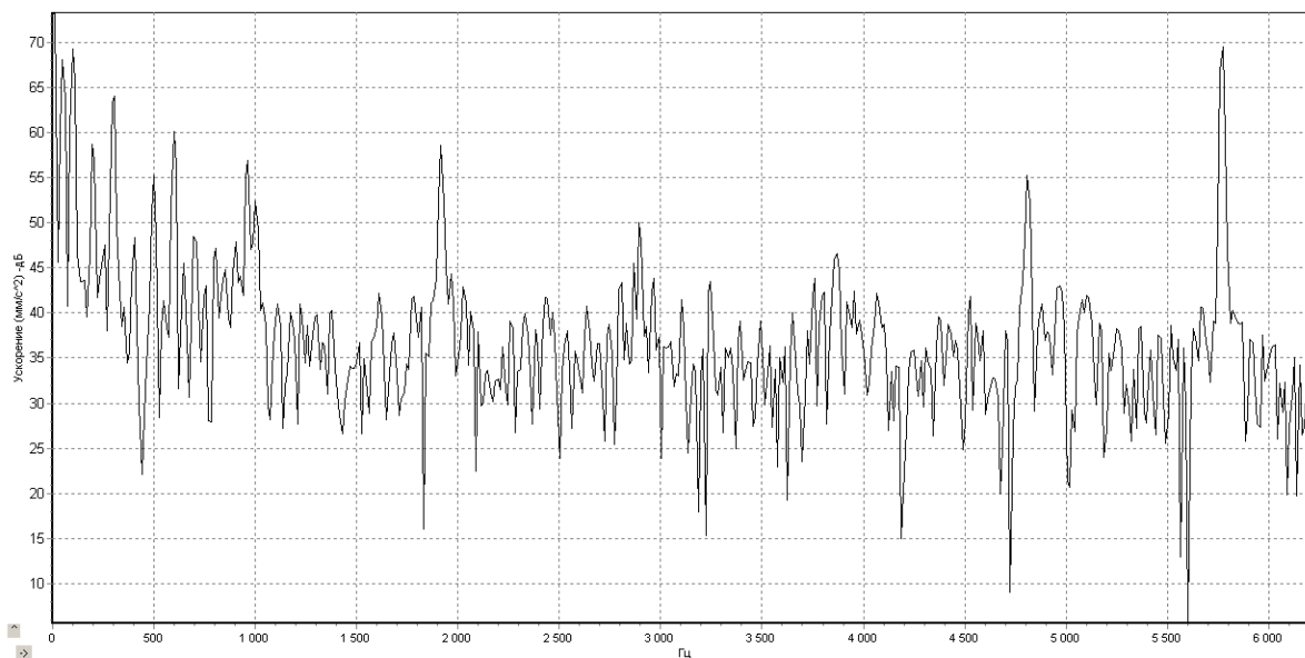
Рис. 4. Вибрация бака трансформатора фирмы «Siemens» на ГПП нефтеперекачивающей станции (фаза С, низкая сторона)
