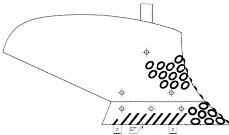
Рис. 3. Расположение прямолинейных и кольцевых валиков твердого сплава в зонах наибольшей интенсивности трения лемешно-отвальной поверхности корпуса плуга с уплотненной почвой [7,8]
