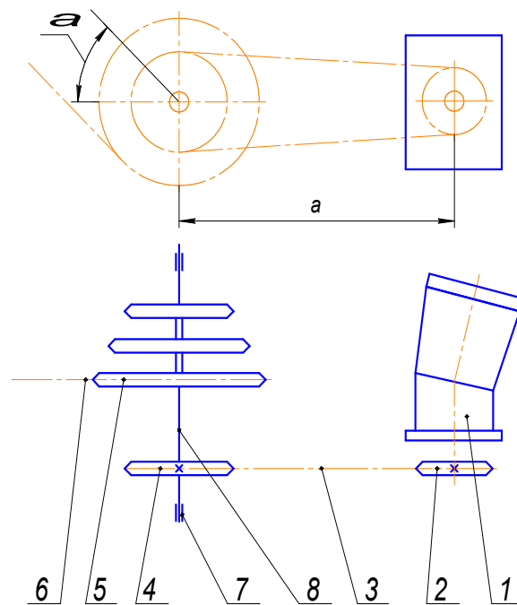
Рисунок 2 – Кинематическая схема привода валов зерно- и туковысевающих аппаратов агрегата АУП-18.
