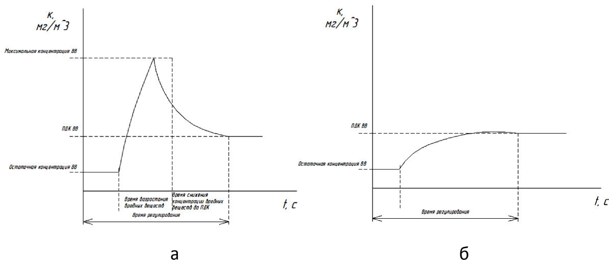
Рис. 2. Изменение концентрации вредных веществ: а) в стандартной системе; б) в предлагаемой системе
