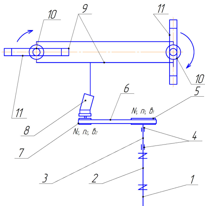
Рис. 1. Кинематическая схема привода рабочих органов косилки.
