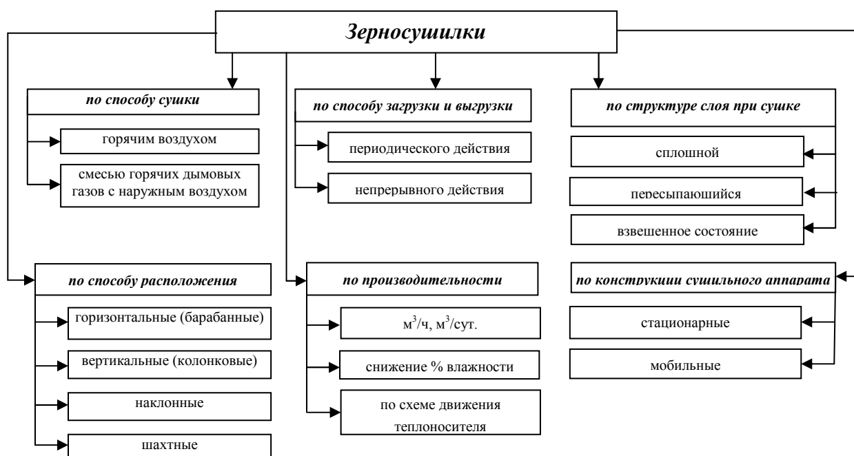
Рис. 2. Классификация зерносушилок
