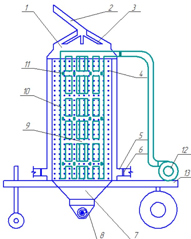
Рис. 3. Малогабаритная зерносушилка
