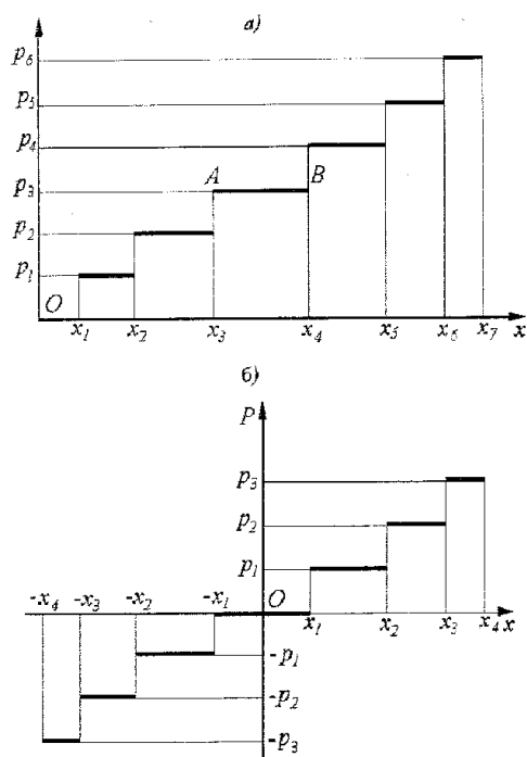
Рис. 2. Универсальная силовая характеристика виброзащитного устройства
