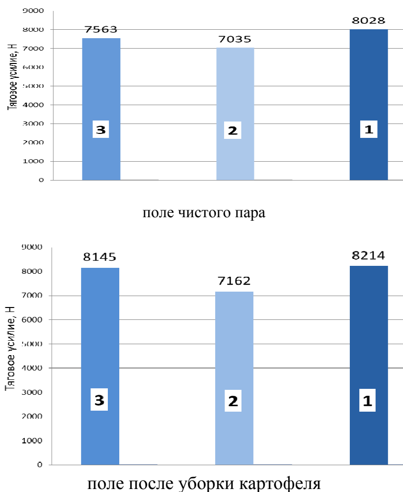
Рис. 7. Средние значения тягового сопротивления навесного плуга ПЛН-3-35 при обработке суглинистой почвы: 1 – лемеха в состоянии поставки с наплавкой тыльной стороны по технологии РЗЗ; 2 – лемеха с наплавкой лицевой поверхности поперечными валиками; 3 – лемеха с наплавкой лицевой поверхности кольцевыми валиками
