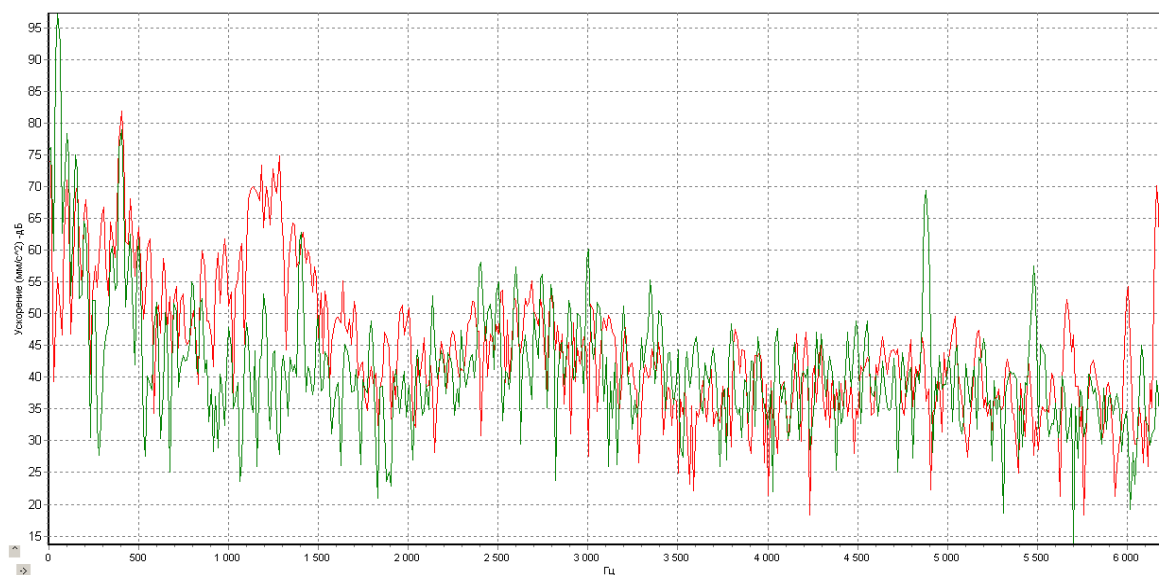
Рис. 5. Вибродиагностирование трансформатора ТЗ подстанции металлургического завода (фаза – С, середина, низкочастотным датчиком, зеленым – 1-ое измерение, красным – 2-ое измерение)
