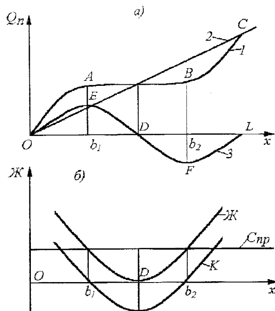
Рис. 1. Характеристики виброзащитного устройства с перескоком: а – силовые характеристики; б – жесткостные характеристики.
