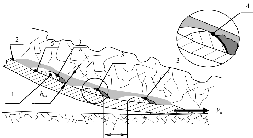
Рис. 2. Схема взаимодействия контактного слоя почвы с рабочей поверхностью детали: V_n – скорость перемещения детали; h_{cl} – толщина контактного слоя почвы; t – шаг наплавки износостойкого материала; 1 – поперечное сечение наплавленного слоя; 2 – поверхность основного металла; 3 – область торможения и смятия контактного слоя почвы; 4 – переходная зона резания и скалывания частиц; 5 – зона застоя почвы на основном металле
