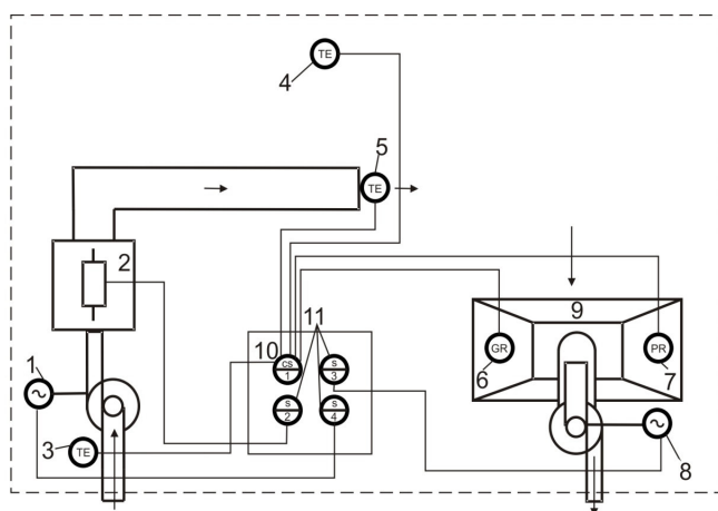
Рис. 1. Функционально-технологическая схема системы вентиляции сварочного цеха
