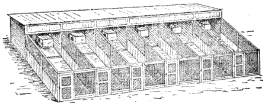
Рис. 1. Навес с выгулами
