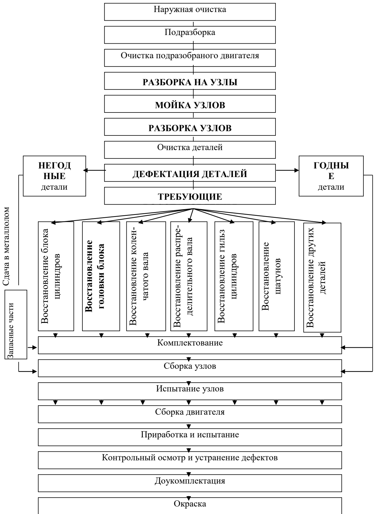
Рисунок 1.2 - Структурная схема технологического процесса капитального ремонта двигателей на мотороремонтном заводе
