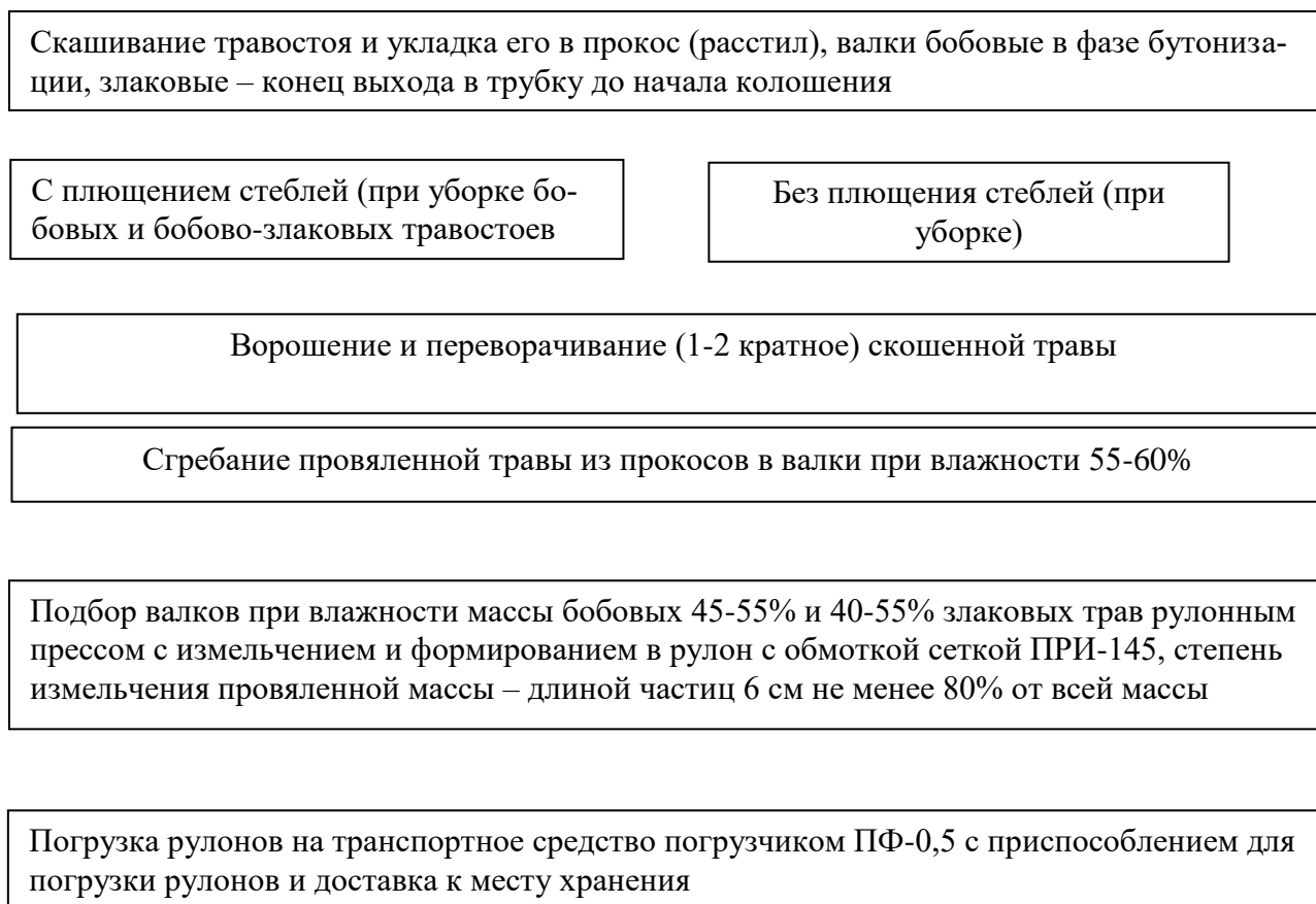
Рис. 2. Схема основных производственных операций технологии заготовки сенажа в рулонах с хранением в полимерном рукаве
