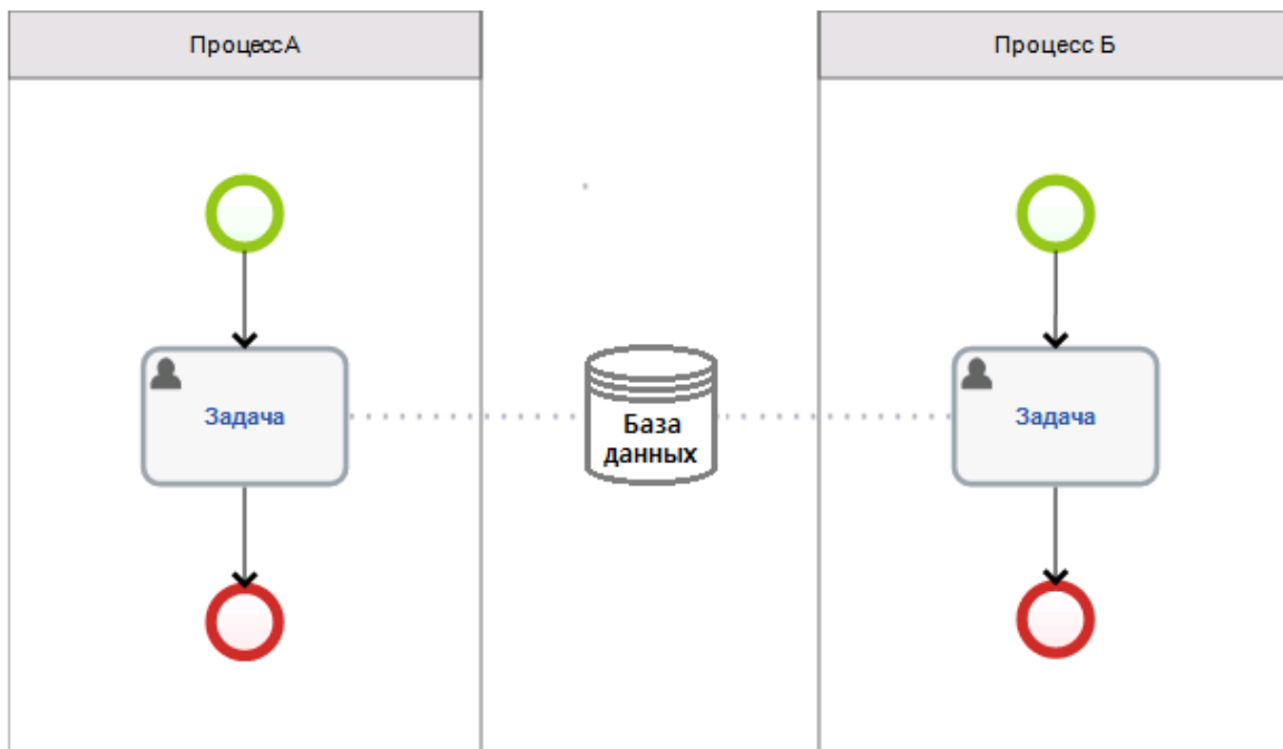
Рис. 34. Межпроцессное взаимодействие через данные
