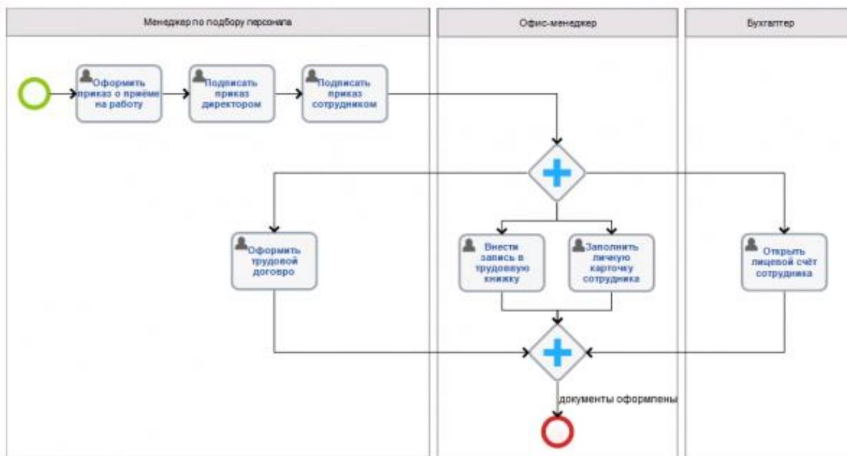
Рис. 10. Подпроцесс «Оформление документов»
