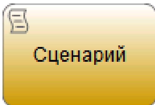
Рис. 5.4. Задача-сценарий
