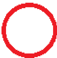
Рис. 1.2. Конечное событие
