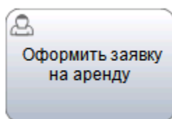
Рис. 1.3. Пользовательская задача
