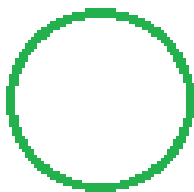
Рис. 1.1. Стартовое событие
