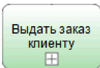
Рис. 6. Задача – Подпроцесс
