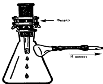
Рис. 50. Фильтр Зейтца и колба Бунзена для фильтрации воды
