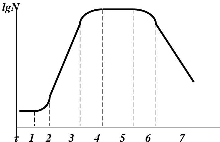
Рис. 25 – Кривая роста статической культуры: N – концентрация жизнеспособных клеток; \tau – продолжительность культивирования
