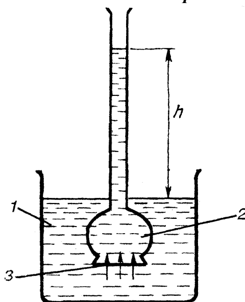
Схема осмометра
