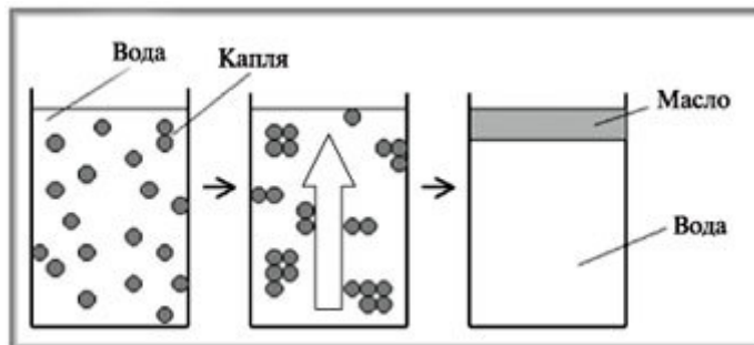
Схема коалесценции и всплывания масла
