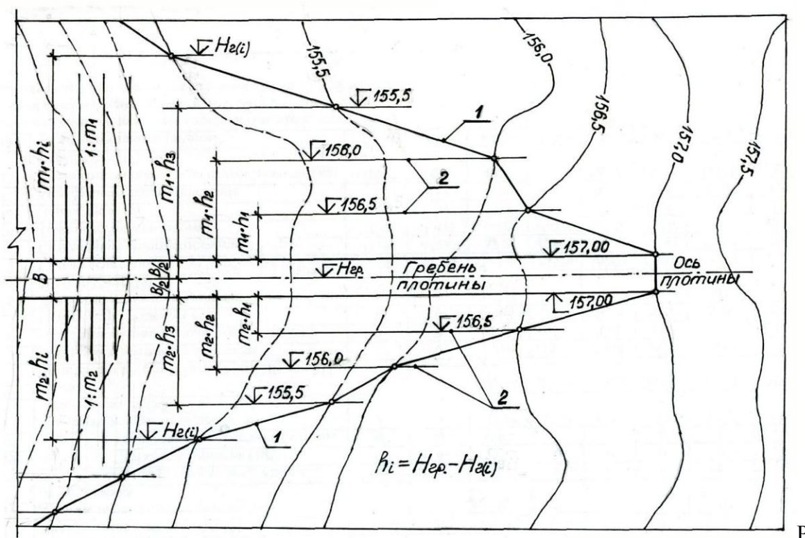
ис. 4.1 Графическое построение линии сопряжения подошвы плотины с поверхностью земли (1-- контур основания плотины; 2 -- соответствующие горизонтали сооружения (откосов плотины) и их высоты ( H_2 ))
