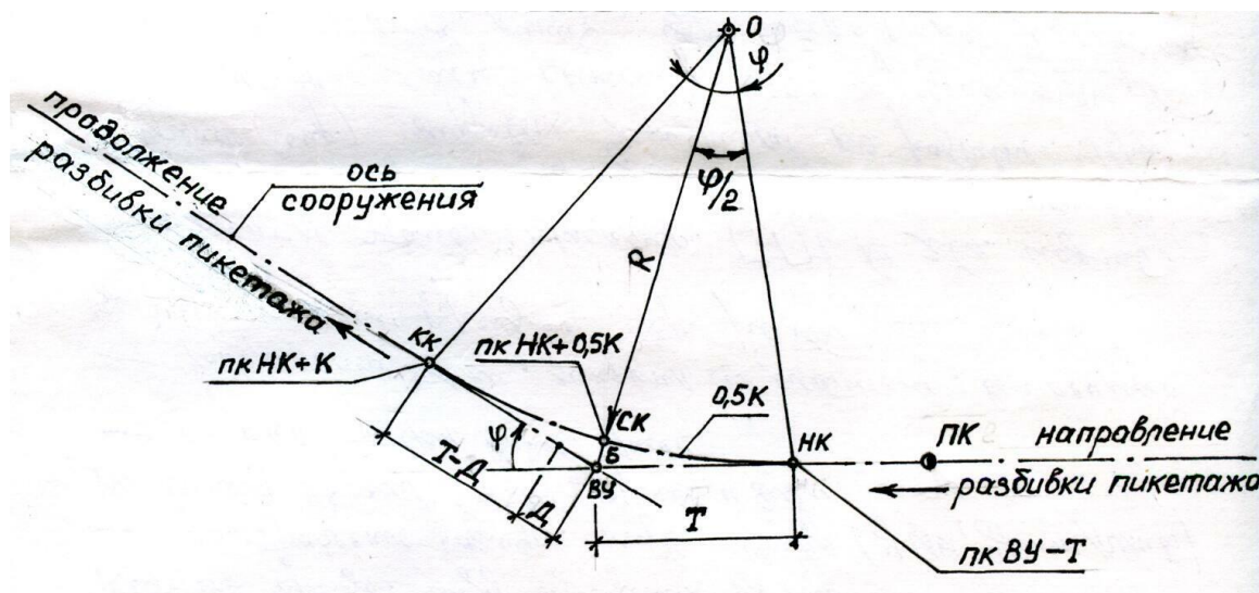
Рис. 3.1 Разбивка пикетажа на криволинейном участке трассы
