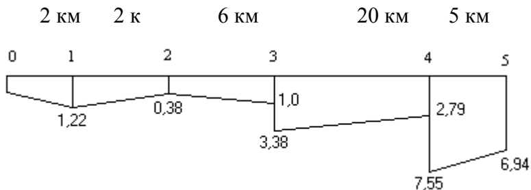
Рис.4.1 Распределение концентраций азота по длине реки, мг/л.
